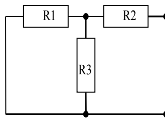
Рисунок 1.2 - Еквівалентна вимірювальна схема
