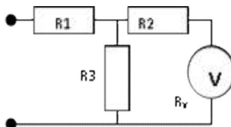
Рисунок 1.1 - Вимірювальна схема
