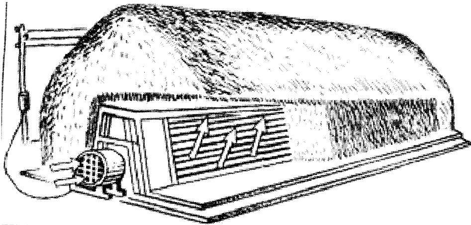
Рис. 42. Досушування сіна в скирті примусовим вентиляванням
