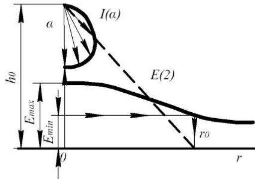
Рис. 12 – Розподіл ІЧ опроміненості на горизонтальній поверхні під опромінювачем
