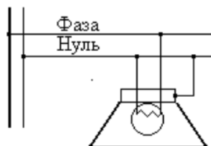
Рис. 3 – Схема заземлення корпусу світильника
