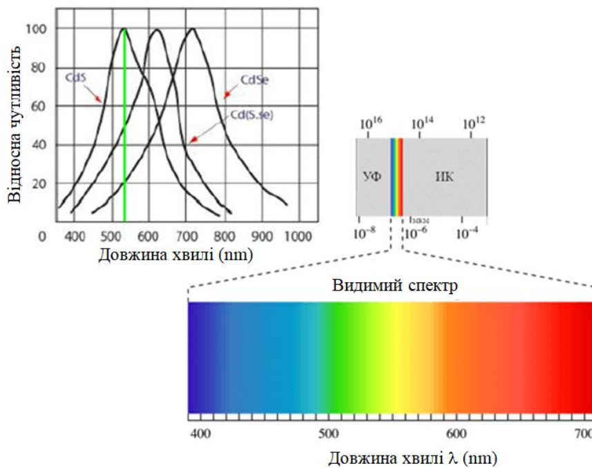
Рис. 8 – Спектри чутливості фоторезисторів
