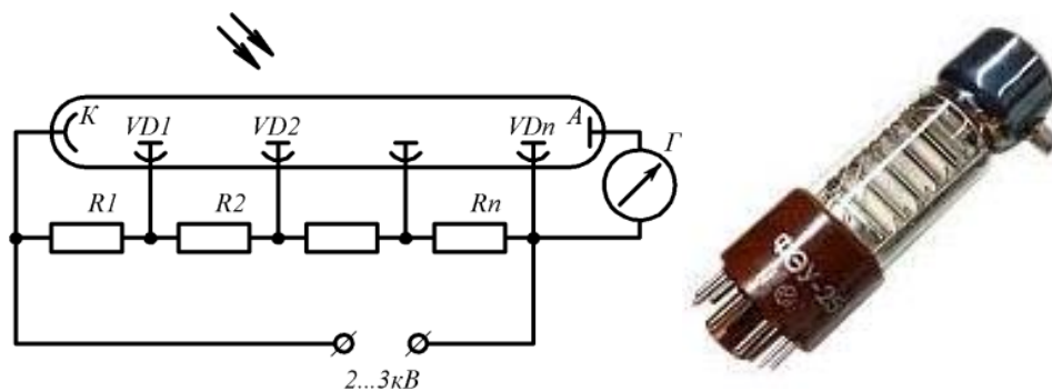
Рис. 14 – Принципова схема вмикання фотоумножувача: К – катод; VD1...VDn – діоди; А – анод; R1...Rn – резистори дільника; Г - вимірювальний прилад, гальванометр.
