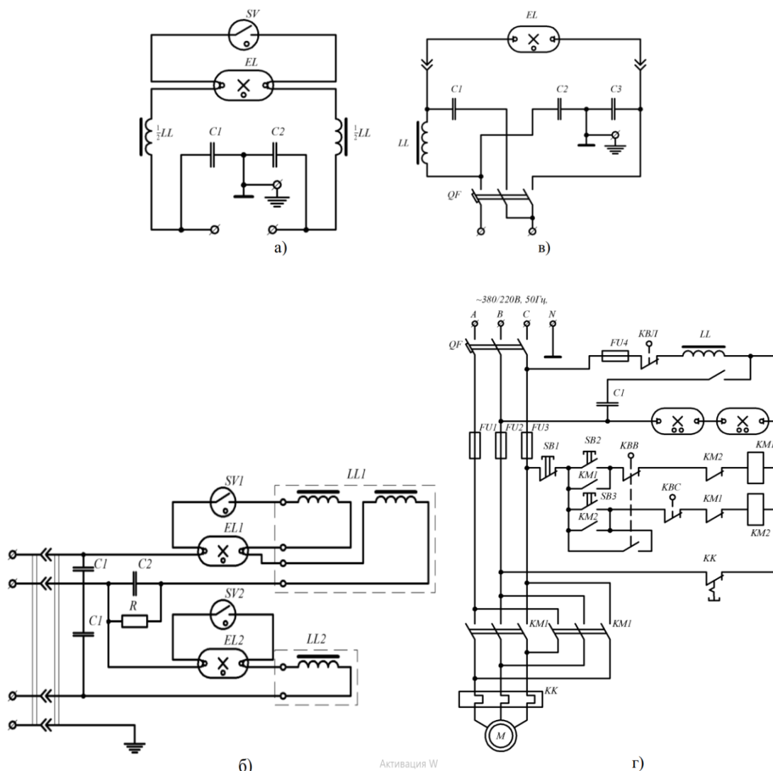
Рис. 3 – Схеми електричні принципи: а) опромінювача EO1-30M; б) світильника-опромінювача ОЕСП02-2×40/П5'X-01; в) опромінювача ртутно-кварцового ОРК-2; г) установки УОК-1.
