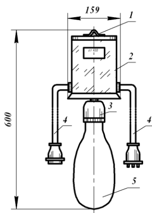
Рис. 2 – Тепличний опромінювач ОТ-400: 1 – вузол підвіски; 2 – ПРА джерела випромінювання; 3 – фарфоровий патрон із ущільнювачем; 4 – кабель живлення опромінювача; 5 – лампа ДРЛФ-400
