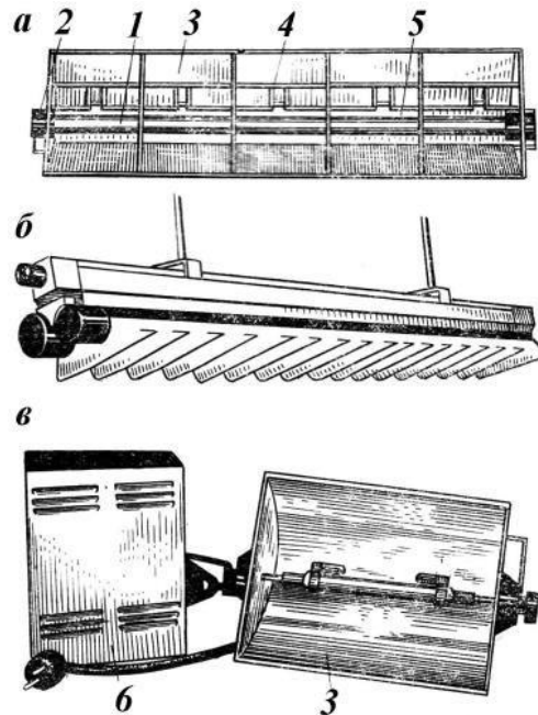
Рис. 2 - Загальний вигляд ультрафіолетових опромінювальних установок: EO1-30M (а), OESP02-2×40/П5'X-01 (б) і ОРК (в); 1 - вітальна лампа; 2 - лампотримач; 3 - відбивач; 4 - захисна сітка; 5 - пуско-регулююча апаратура; 6-пуско-регулюючий пристрій
