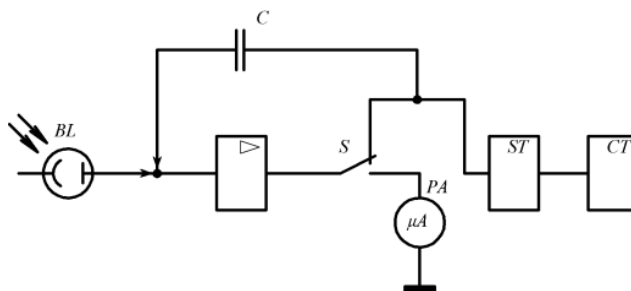
Рис. 23 – Спрощена функційна схема ердозиметра УФД-1А.
