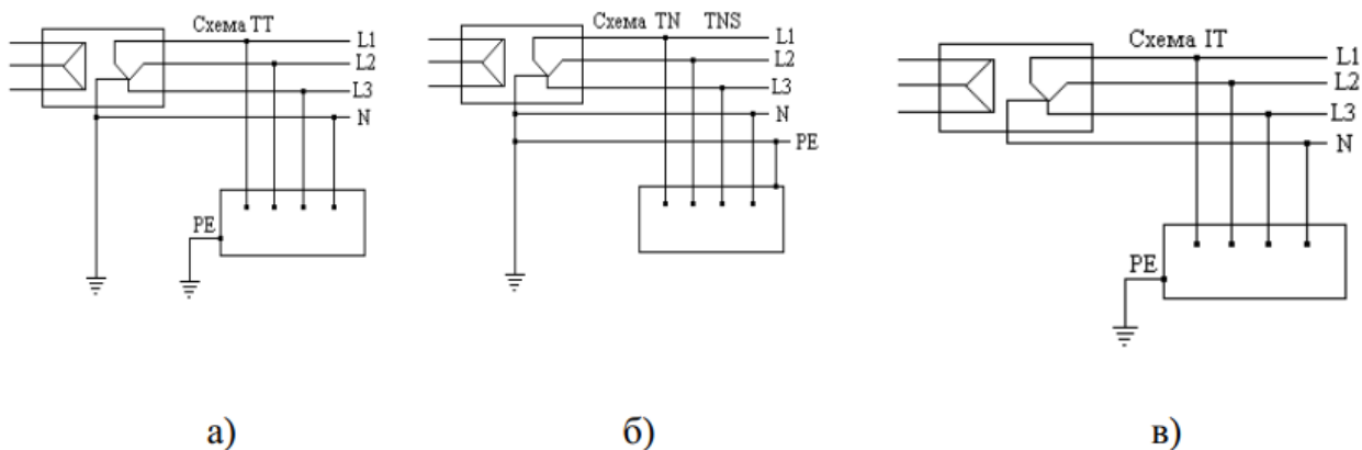
Рис. 2 – Системи заземлення: а) ТТ - нейтраль джерела і корпусу електроприймачів заземлені; б) ТN - нейтраль джерела заземлена а корпуси електроприймачів занулені; в) ІТ - нейтраль джерела ізольований а корпуси електроприймачів заземлені.
