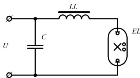
Рис.2 – Принципова схема включення чотириелектродних ламп типу ДРЛ:
