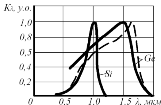
Рис. 11 – Спектри чутливості фотодіодів на основі германія (Ge) і кремнія (Si)
