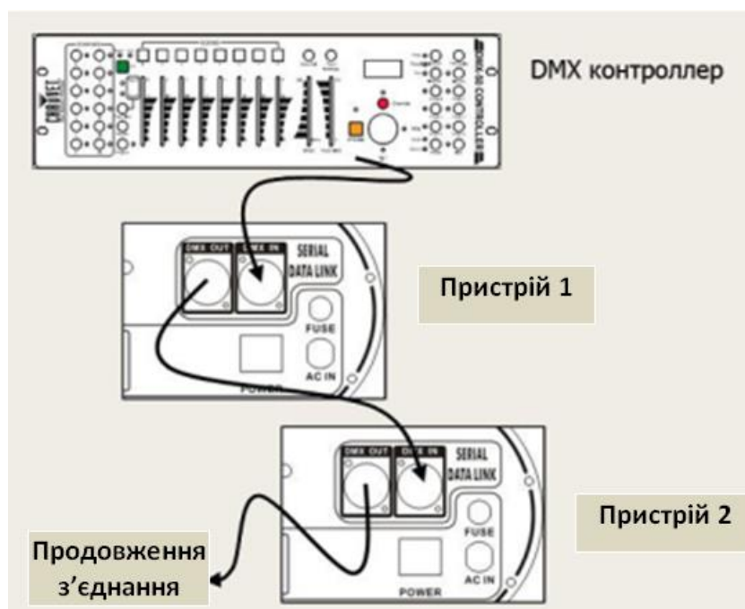
Рис. 3 – Спосіб і порядок підключення декількох світильників до одного контролера
