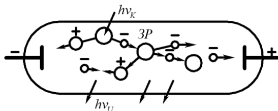
Рис. 1 – Розряд в газі: h\nu_k – зовнішній збудник; h\nu_u – випромінювання розряду; ЗР – збудження в розряді
