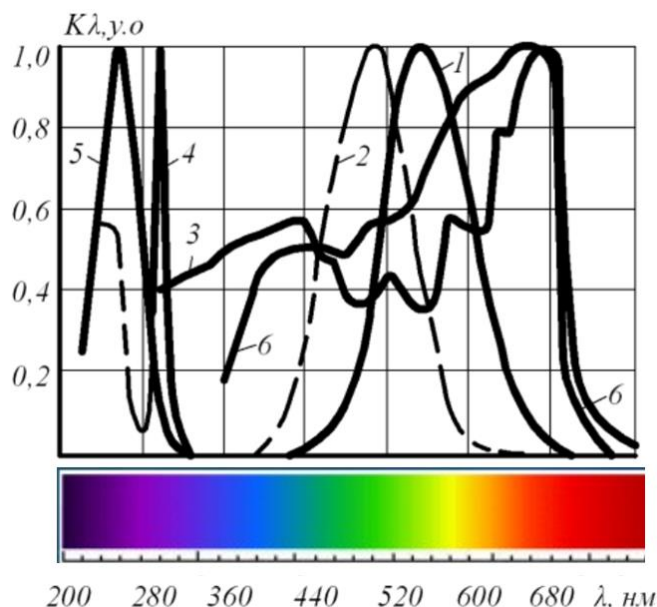
Рис. 5 – Спектральні характеристики: 1 – око людини вдень; 2 – око людини вночі; 3 – зеленого листа по І.І.Свентицькому (теоретична); 4 – шкіра тварини (вітальна); 5 – бактерій; 6 – фотосинтез по Мс. Скрі (експериментальна)
