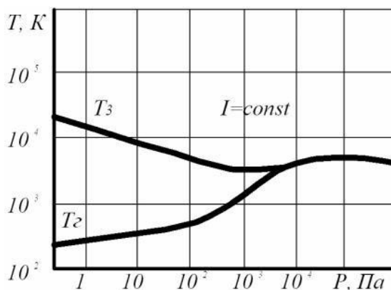
Рис. 2 – Вимірювання температури газу T_g і електронної температури T_e при зміні тиску
