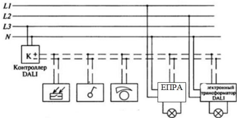
Рис. 2 – Управління освітленням за цифровою схемою
