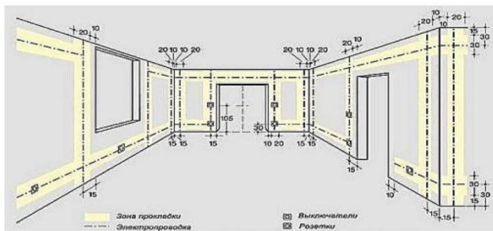
Рис. 2 – Приклад прокладання мережі
