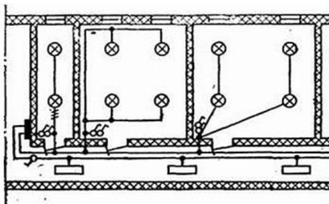
Рис. 1 – Схема компонентування групових мереж
