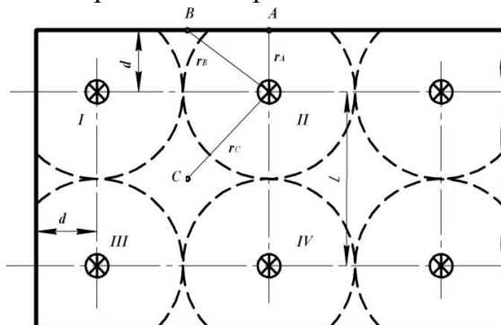
Рис. 7 – Розрахунок опромінюючої установки з точковими випромінювачами: розміщення опромінювачів на плані стелажа і визначення найменших допустимих відстаней між ними
