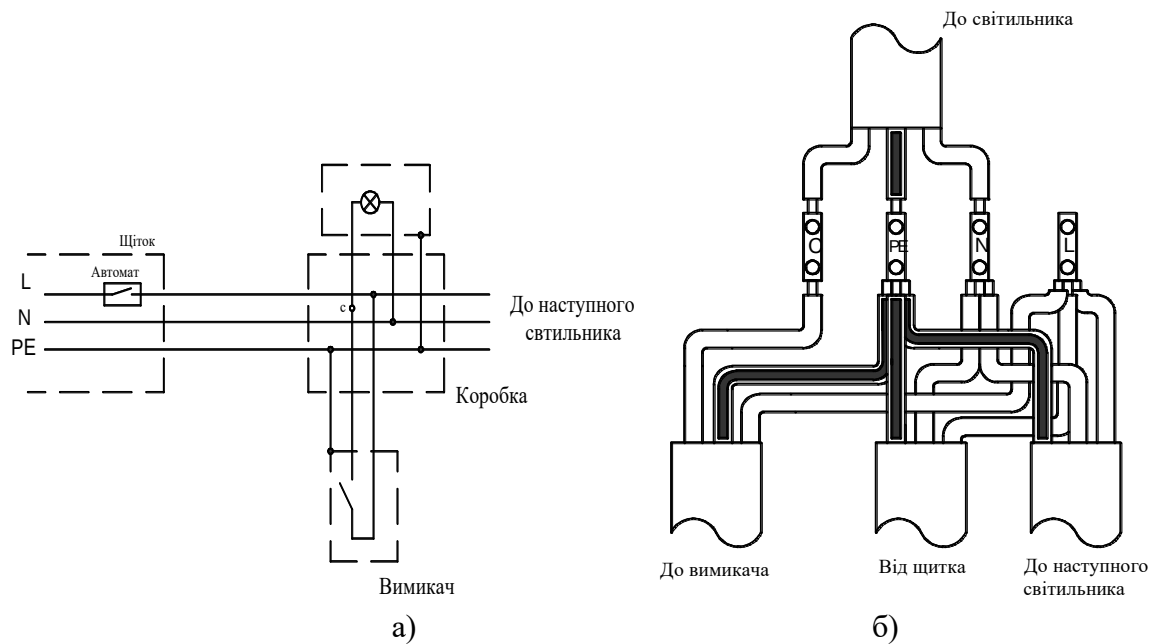
Рис. 2 – Най простіша принципова схема підключення світильника: а) схематичний вид; б) вид на практиці.
