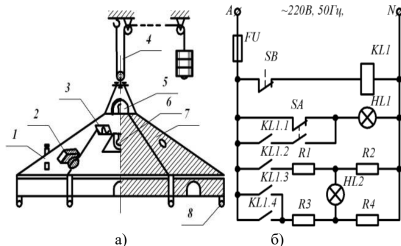
Рис. 11 – Брудер БП-1: а) Загальний вигляд; б) Принципова електрична схема брудера БП-1: 1 – контрольний термометр; 2 – терморегулятор; 3 – ІЧ-опромінювач; 4 – тросова підвіска з противагами; 5 – сигнальна лампа перегорання ТЕНів; 6 – лампа освітлення; 7 – корпус; 8 – упори.
