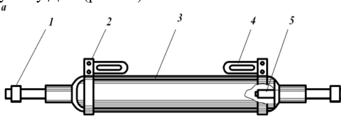
Рис. 10 – Конструкція лампи ДРТ: 1 – ввід; 2 – металеві хомутки; 3 – трубка із кварцового скла; 4 – тримачі; 5 – електроди;
