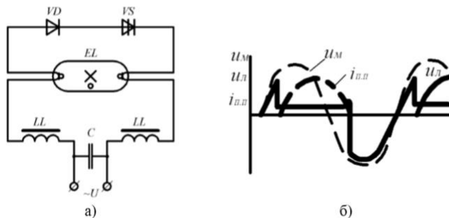
Рис. 10 – а) Схема включення ЛЛ з напівпровідниковим стартером; б) Осцилограми миттєвих значень напруги і струму при запалюванні люмінесцентної лампи за допомогою динистора. VS - динистор; VD – діод; LL – дросель; EL – люмінесцентна лампа
