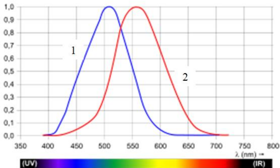
Рис. 3 – Середнє значення спектральної чутливості ока: 1 - усереднена крива спектральної чутливості ока; 2 - крива спектральної чутливості ока в умовах нічного зору.
