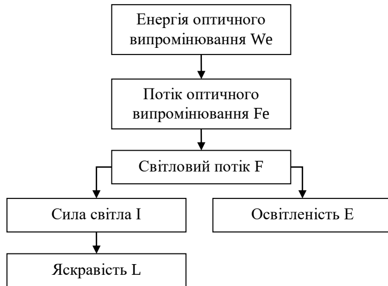
Рис. 1. – Енергетичні величини оптичного випромінювання
