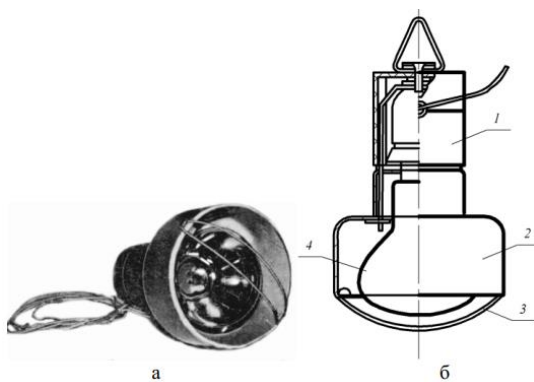
Рис. 8 – Опромінювач ветеринарний типу ОВИ-1: а) загальний вигляд; б) розріз: 1 – корпус; 2 – пластмасовий ковпак; 3 – захисна сітка; 4 – ІЧ-лампа
