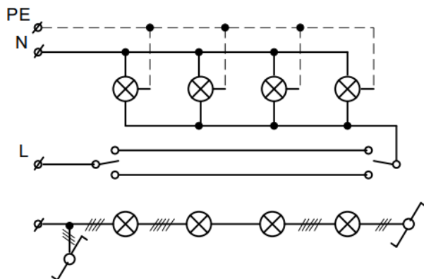
Рис. 6 – Коридорна схема управління освітленням
