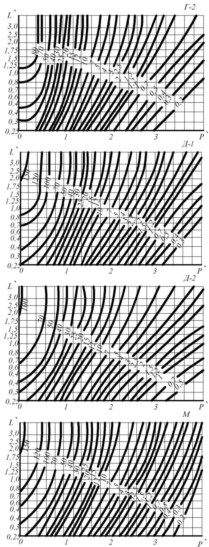
Рис. 2 – Криві рівної освітленості для світлових ліній з найбільш розповсюдженими світильниками з люмінесцентними лампами і різними повздовжніми деталізованими кривими сили світла \Gamma-1 , \Gamma-2 , D-1 , D-2 , M
