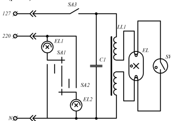
Рис. 3 – Електрична принципова схема випромінювача ІКУФ-1
