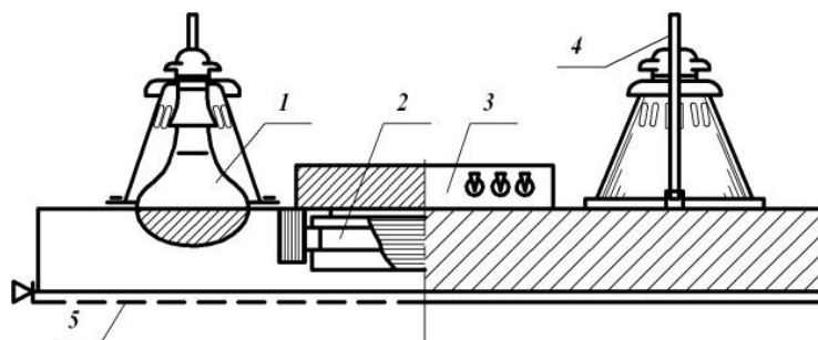
Рис. 2. – Конструкція опромінювальної установки ІКУФ-1: 1 – ІЧ-лампа; 2 – вітальна лампа; 3 – кожух ПРА з перемикачами; 4 – підвіска; 5 – захисні решітки
