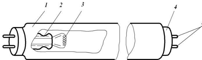
Рис. 6 – Конструкція люмінесцентної лампи загального призначення в розрізі
