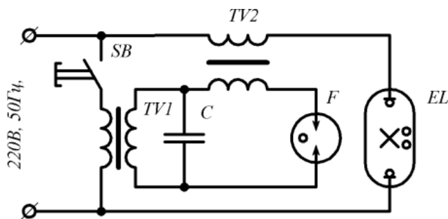
Рис.4 – Схема включення лампи ДРІ
