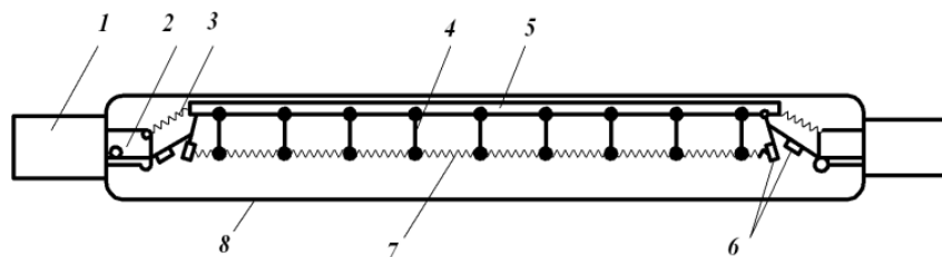
Рис. 9 – Конструкція трубчастого ІЧ випромінювача: 1- цоколь; 2 – штангель; 3 – пружина, яка підтримує стержень; 4 – молібденові тримачі; 5 – скляний стержень; 6 – електроди; 7 – вольфрамові тіла розжарювання; 8 – скляна трубка.
