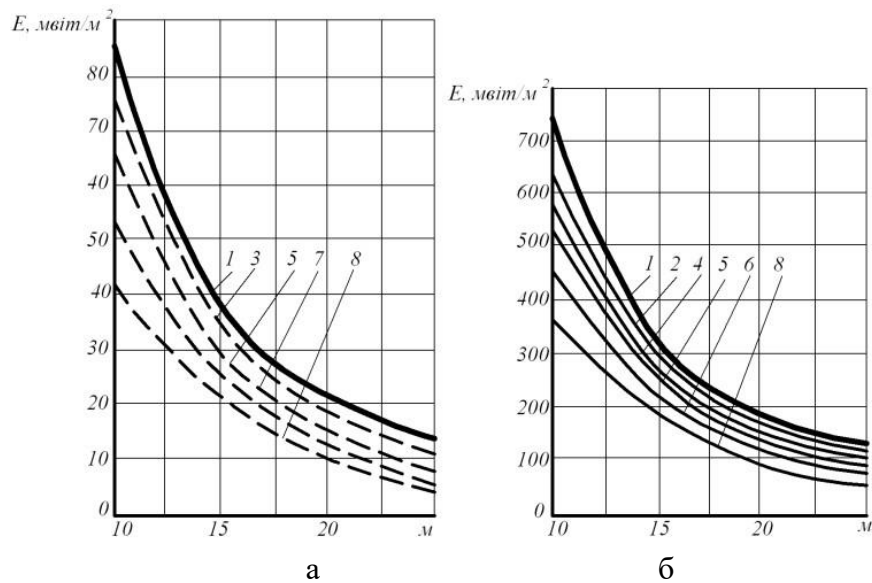
Рис. 8 - Залежність вітальної опроміненості, створюваної лампою ЛЕ30-1 (а) і ДРТ400 (б), від відстані до опромінювальної поверхні та тривалості горіння ламп: 1 - нова лампа; 2 - після 100 год. експлуатації; 3 - після 150 год.; 4 - після 200 год.; 5 - після 300 год.; 6 - після 500 год.; 7 - після 600 год.; 8 - після 1000 год. експлуатації
