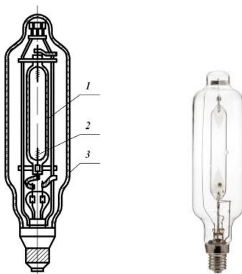
Рис. 3 – Будова лампи ДРИ
