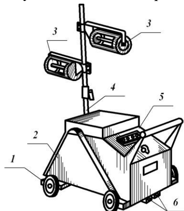
Рис. 7 – Установка для опромінення птиці УОК-1: 1 – самохідне шасі; 2 – привод від електродвигуна до ведучих коліс і пристрою укладки кабелю; 3 – опромінювачі з
