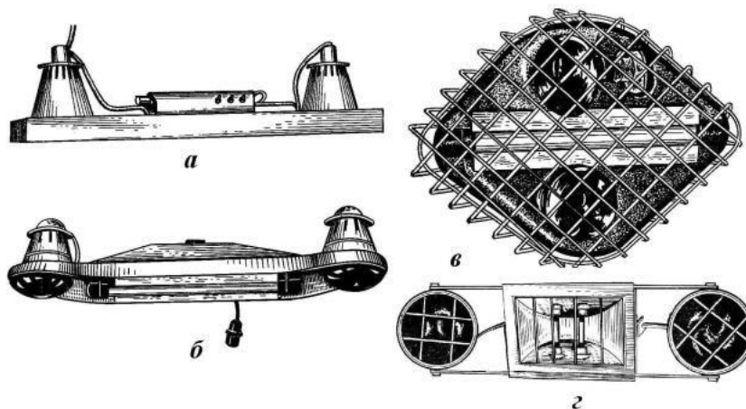
Рис. 1 – Загальний вигляд опромінювачів автоматизованих установок інфрачервоного обігріву та ультрафіолетового опромінення молодняка тварин та птиці: а) ІКУФ-1; б) ІКУФ-1М; в) «Луч»; г) СОЖ-1
