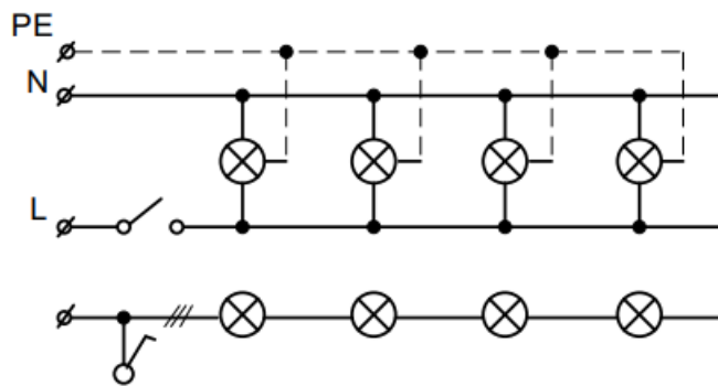
Рис. 2 – Схема включення ламп одним вимикачем
