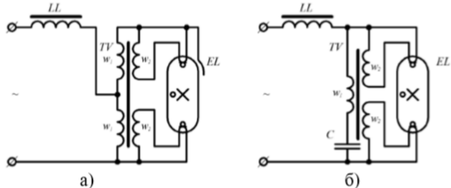
Рис. 11 – а) Безстартерна схема включення ЛЛ з розжарювальним трансформатором гарячого запалювання: EL – люмінесцентна лампа; LL – дросель; TV - розжарювальний трансформатор; б) Резонансна безстартерна схема включення ЛЛ з розжарювальним трансформатором холодного запалювання: C – конденсатор; w1 – первинна обмотка трансформатора; w2 – вторинна обмотка трансформатора
