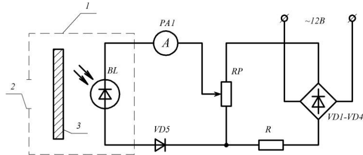
Рис. 10 – Схема вимірювача опроміненості з фотодіодом: BL - фотодіод ФД-6Г; RP - потенціометр; PA1 - мікроамперметр; R – обмежувачий опір; VD1...VD4 - випрямний міст; VD5 - блокуючий діод; 1 - корпус вимірювача; 2 – вікно; 3 - світлофільтр.
