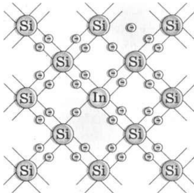
Ковалентний зв'язок
