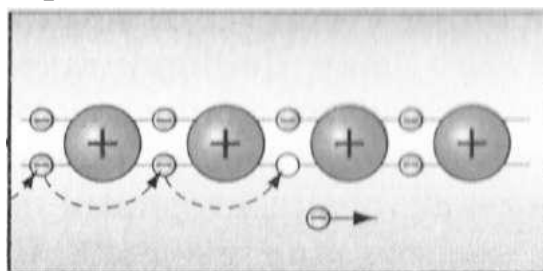
Діркова провідність
