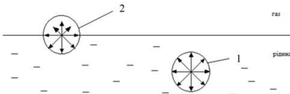
Рис. 3.1 Схема дії міжмолекулярних сил усередині рідини й на її поверхні.
