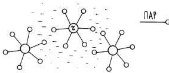
Рис. 2.1. Стабілізація колоїдної системи за допомогою ПАР
