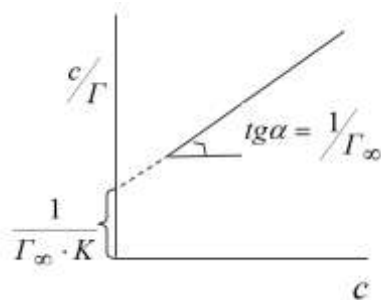
Рис. 4.3. Ізотерма адсорбції Ленгмюра в прямолінійних координатах.
