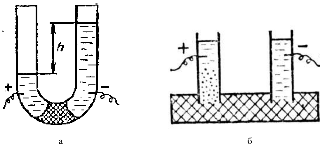
Рис. 7.6. Схеми дослідів Рейсса.
