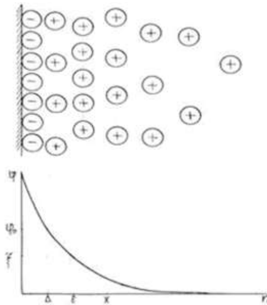
Рис. 7.3. Схема будови подвійного електричного шару і крива зміни потенціалу.
