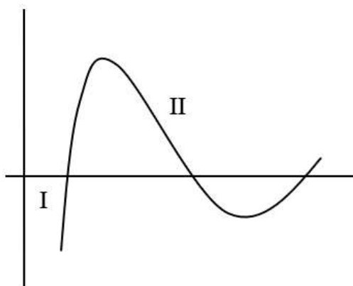
Рис. 9.1. Потенційна крива взаємодії двох колоїдних часток.
