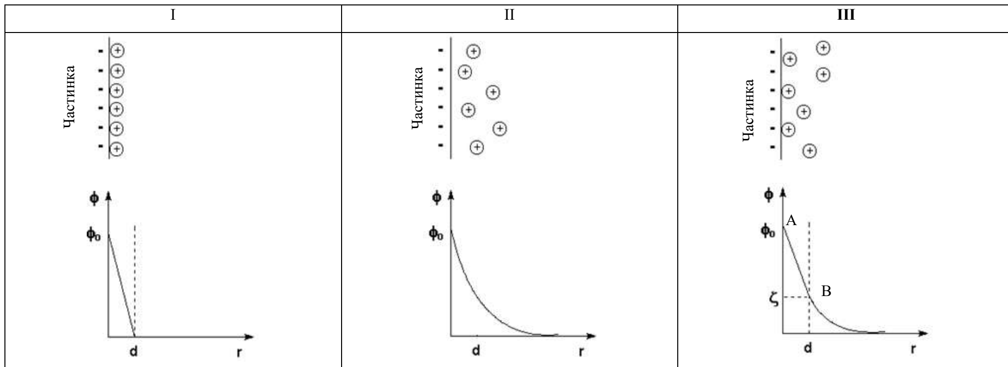
Рис. 7.2. Будова подвійного електричного шару:
