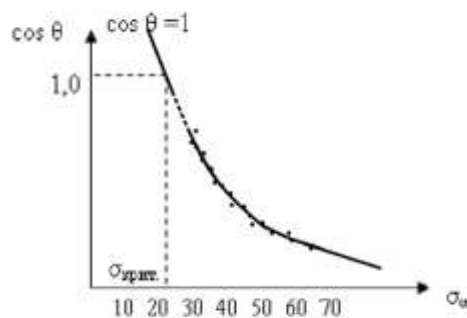
Рис. 3.4. Визначення \sigma_{тв.т.} за Зисманом
