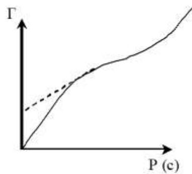
Рис. 4.6. Ізотерма полімолекулярної сорбції.
