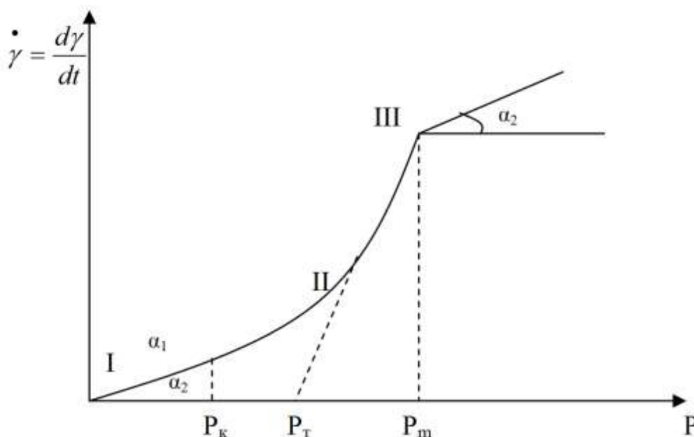
Рис. 9.4. Крива плинності псевдопластичної рідини.
