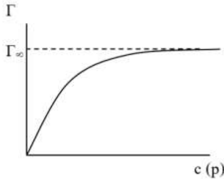
Рис. 4.2. Ізотерма адсорбції Ленгмюра
