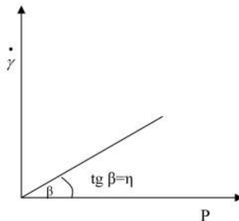
Рис. 9.2. Залежність між швидкістю деформації й напругою зрушення.
