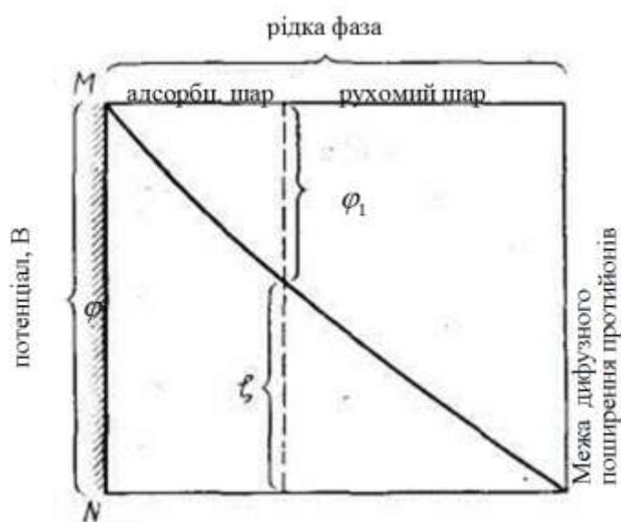
Рис. 7.4. Падіння потенціалів в подвійному електричному шарі.
