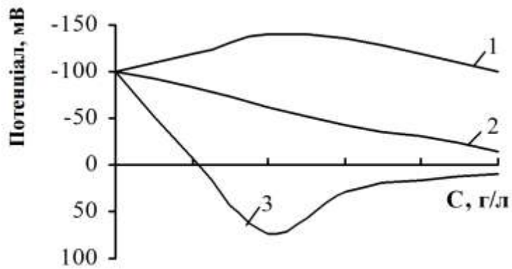
Рис. 7.5. Залежність електрокінетичного потенціалу від концентрації електроліту для одно- (1), дво- (2) і три- (3) зарядних протийонів.
