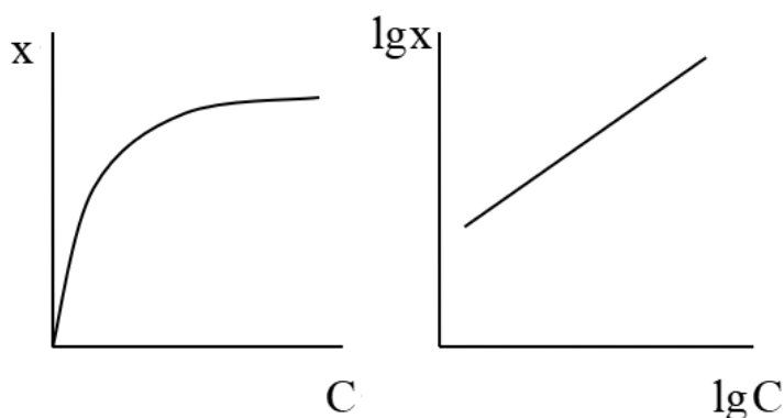
Рис. 4.5. Ізотерми адсорбції Фрейдліха.
