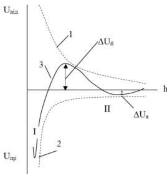
Рис. 6.3. Потенційні криві взаємодії колоїдних частинок:
