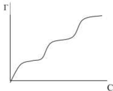
Рис. 4.4. Ізотерма східчастої адсорбції.
