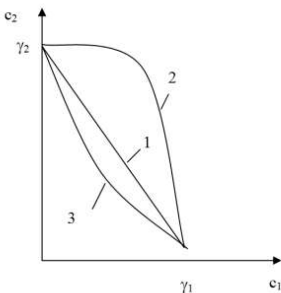
Рис. 6.2. Спільна дія електролітів при коагуляції.
