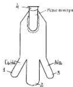
Рис. 2.2. Схема приладу Рогінського і Шальнікова
