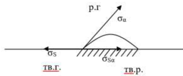
Рис. 3.3. Дія трьох сил ПН.
