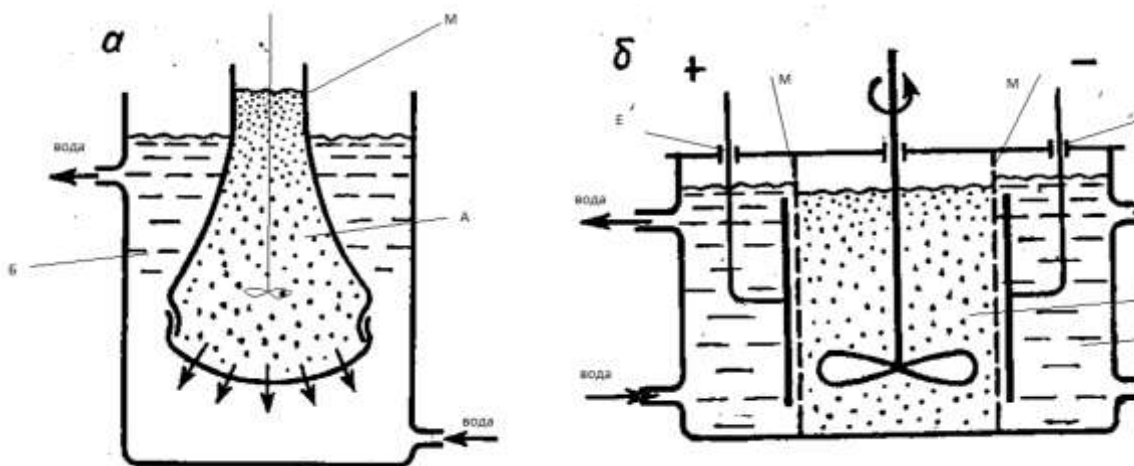
Рис. 2.3. Схеми діалізатора (а) і електродіалізатора (б)
