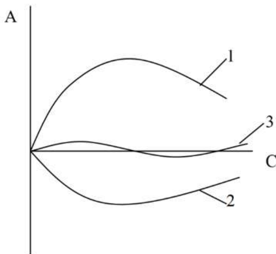
Рис. 5.5. Залежність адсорбції від концентрації адсорбтива:
