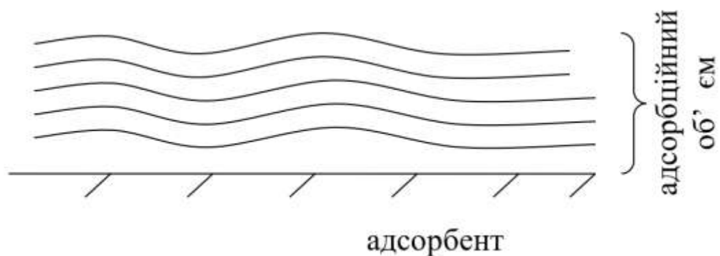
Рис. 4.7. Схема адсорбційного об'єму.
