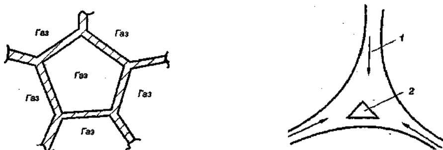
Рис. 10.1. Схема будови піни:
