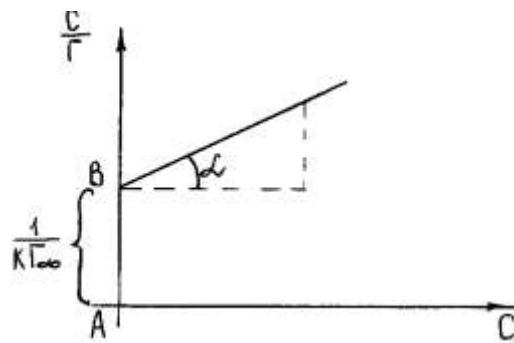
Рис. 5.4. Графік рівняння Ленгмюра в прямолінійних координатах.
