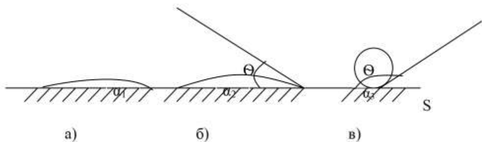
Рис. 3.2. Контактні кути, утворені рідинами на поверхні твердого тіла:
