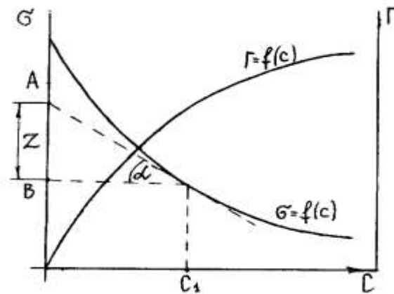
Рис. 5.3. Побудова ізотерми адсорбції за ізотермою поверхневого натягу.
