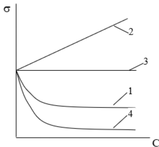
Рис. 5.1. Залежність поверхневого натягу від концентрації розчину:
