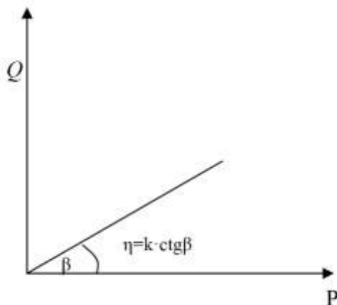
Рис. 9.3. Залежність витрат рідини від тиску.
