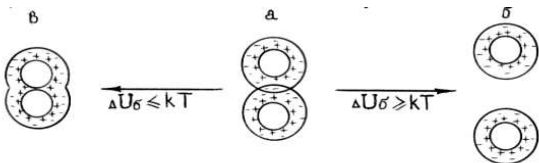
Рис. 6.5. Схеми взаємодії колоїдних часток.
