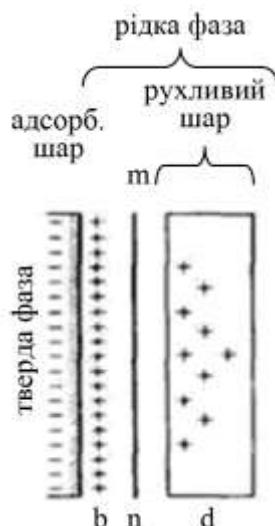
Рис. 7.1. Схема розташування зарядів біля поверхні твердої частинки.
