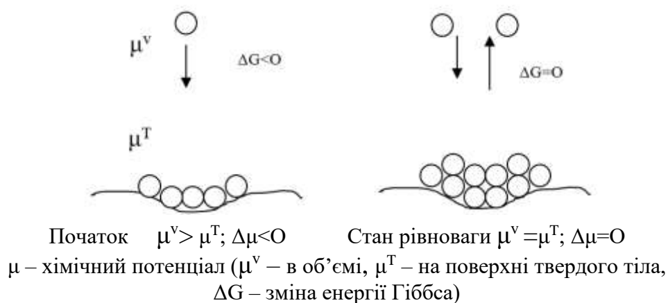
Рис. 4.1. Схеми адсорбції.
