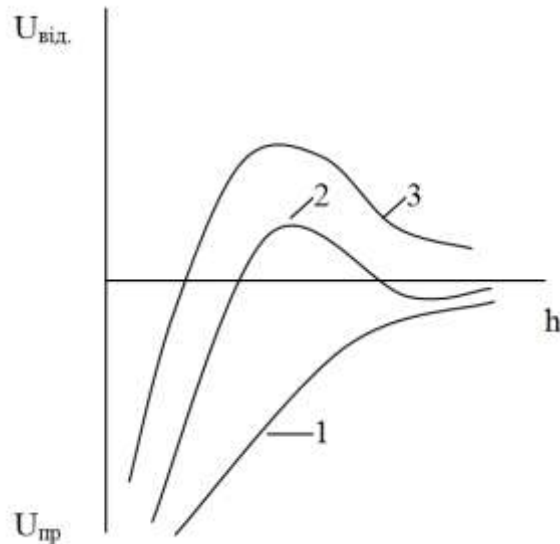
Рис. 6.4. Потенційні криві для певних станів стійкості дисперсної системи:
