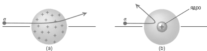
Рис. 36 .Розсіяння \alpha -частинок в атомі Томсона (а) і в атомі Резерфорда (b).
