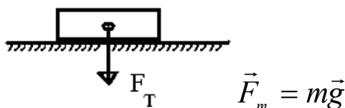
Рис. 2 Сила тяжіння
