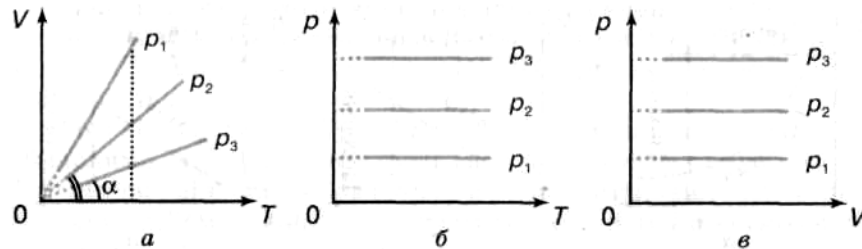
Рис.5. Ізобарний процес
