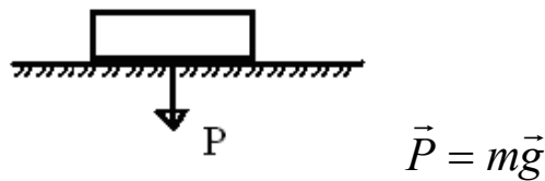
Рис.3 Вага
