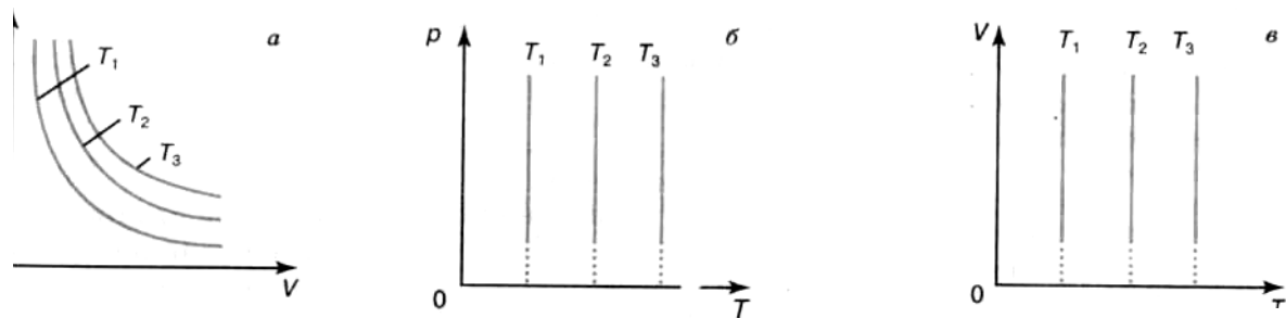
Рис.7. Ізотермічний процес
