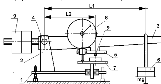
Рис. 2. Схема прибора для определения прочностных характеристик семян
