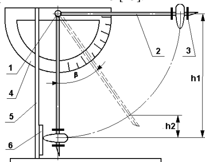
Рис. 1. Схема прибора для определения коэффициента восстановления
