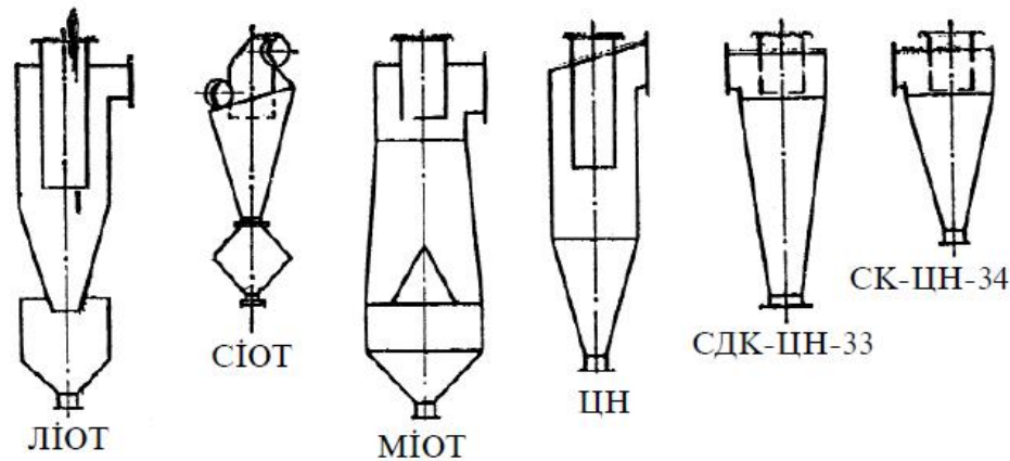
Рис. 5.4. Основні види конструкцій циклонних пиловловлювачів
