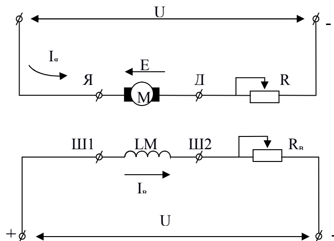
Рис. 2.1 - Схема включення двигуна постійного струму з незалежним збудженням
