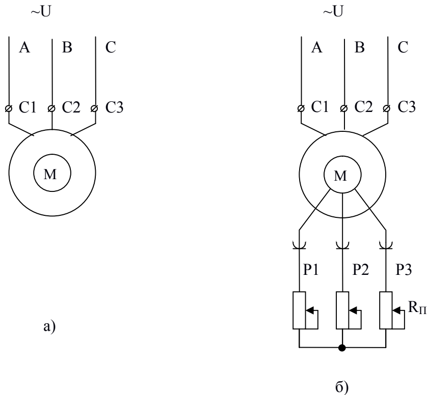
Рис. 2.14. а) схема включення АД з короткозамкненим ротором; б) схема включення АД з фазним ротором.
