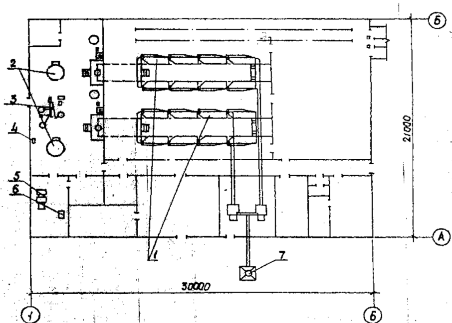
Рис. 3. Доїльно-молочний блок на дві установки УДА-8 типу «Тандем»
