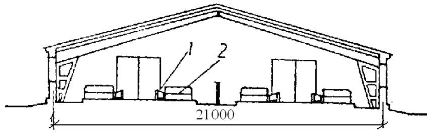
Рис. 2. Схема корівника для безприв'язного утримання тварин з суміщеними місцями відпочинку і годівницями: 1 – годівниця; 2 – бокс для відпочинку корів.
