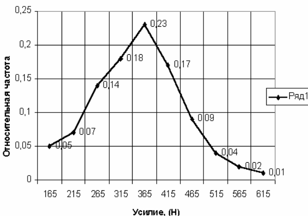
Рис. 3. Варіаційні криві зусиль відокремлення качана від плодоніжки при куті орієнтації 90°:
