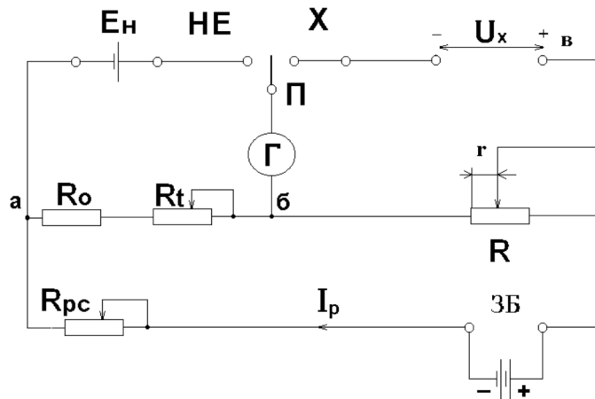
Рисунок 6. Схема компенсатора
