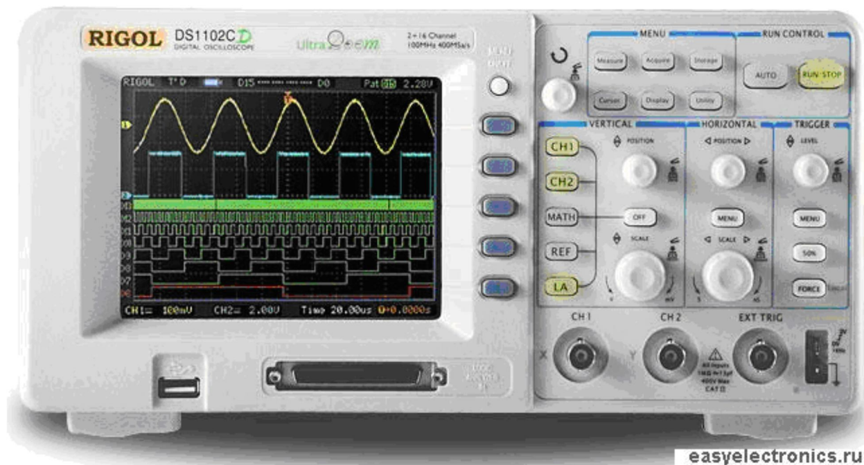
Рисунок 2. Цифровий осцилограф
