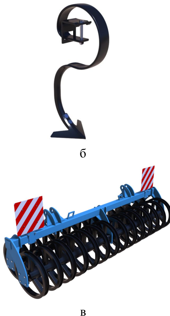
Рис. 5.1. Культиватор причіпний для суцільного обробітку ґрунту МАKTILLER-8:
