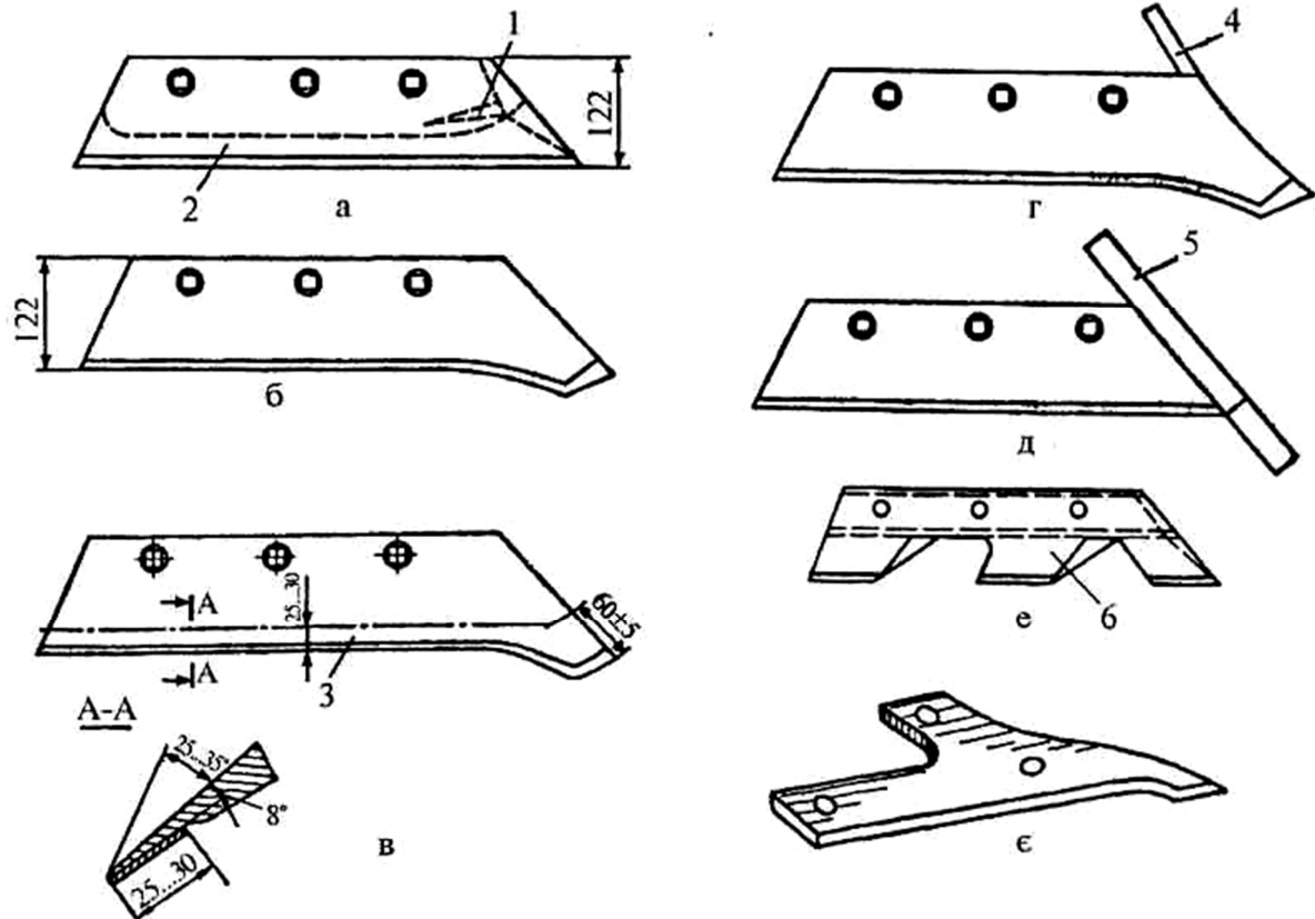
Рис. 1.3. Типи лемешів: а – трапецієподібний; б – долотоподібний; в – долотоподібний з наплавленим твердим сплавом; г – долотоподібний з щогою; д – з висувним долотом; е – трапецієподібний з вирізами; є – вирізний; 1 – магазин; 2, 3 – зони гартування; 4 – щока; 5 – долото; 6 – виступ з потовщенням
