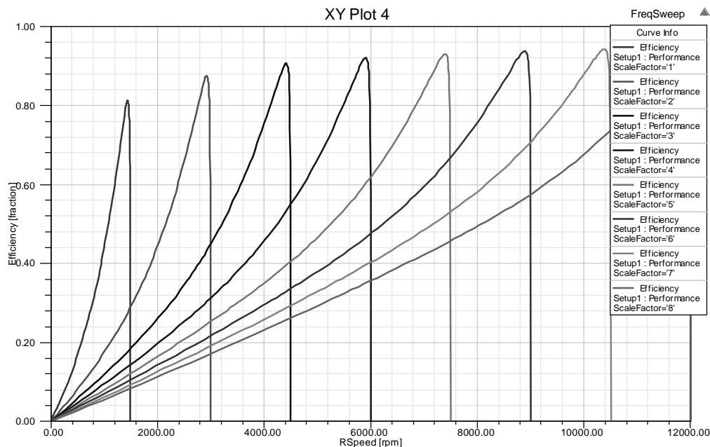
Рис. 7. Сімейство кривих залежності \eta = f(n) ККД \eta (%) електродвигуна від швидкості обертання ротора n (об/хв) при варіаціях частоти f = 50, 100 \dots 400 Гц
