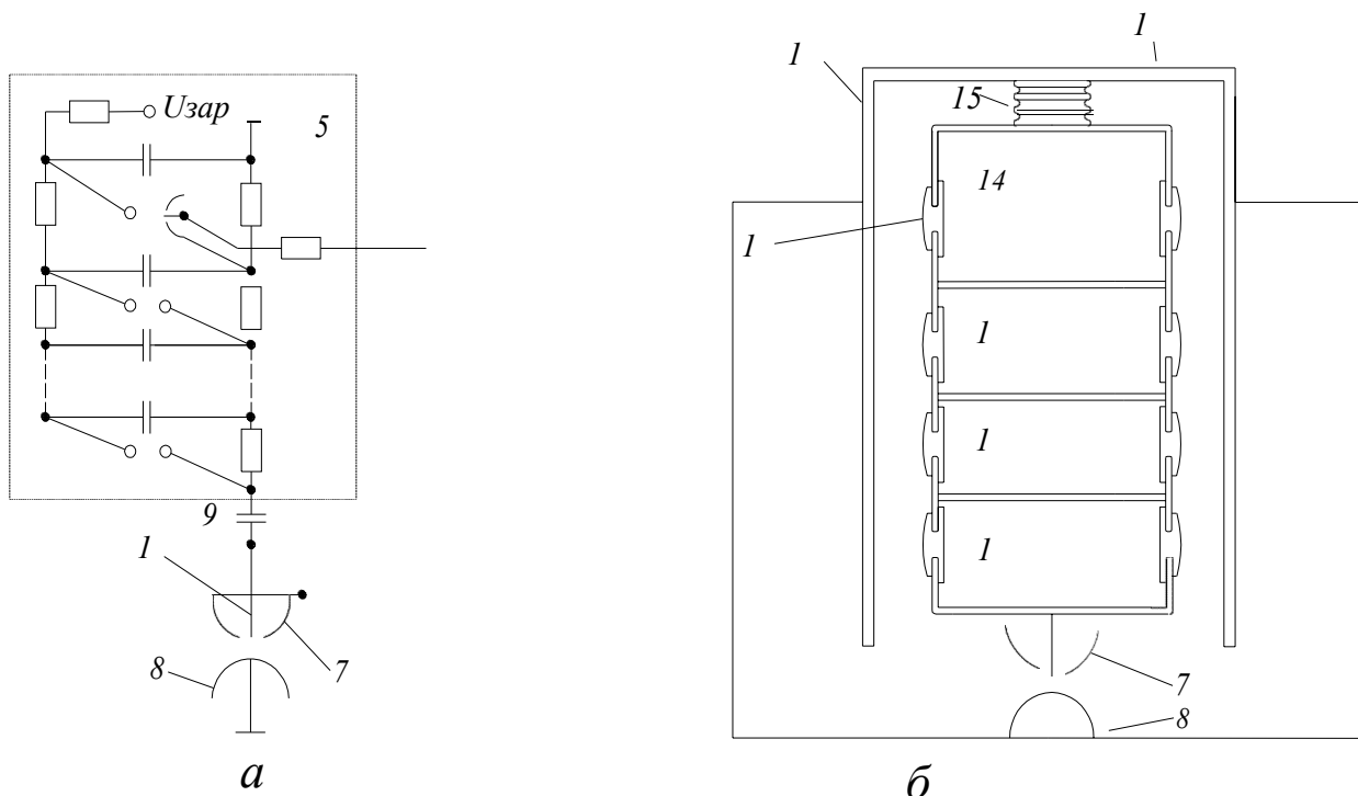
Рис. 4 — Генератор імпульсних напруг за схемою Ірвіна Маркса: а) принципова схема; б) конструкція; U_{zap} — джерело високої напруги;
