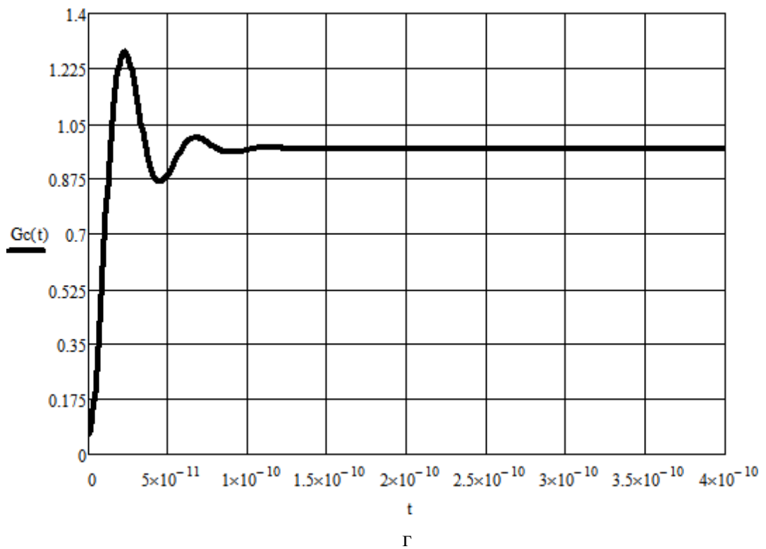
Рис. 9 Розрахункова реакція на прямокутний імпульс спроектованого діляника напруг при значенні опору демпферного резистора R_2 : а – 1 Ом, б –
