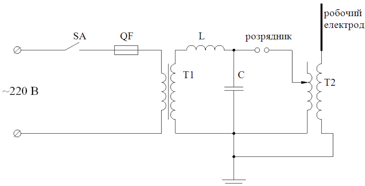
Рис. 12 – Схема електрична принципова лабораторної установки для незараження зернової продукції
