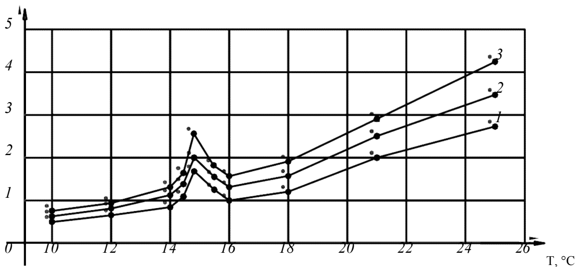
Рис. 2 — Температурна залежність питомої електропровідності зернової маси ячменя сорту "Нева": 1 — напруженість поля 2 кВ/см; 2 — напруженість поля 2,66 кВ/см; 3 — напруженість поля 3,33 кВ/см.
