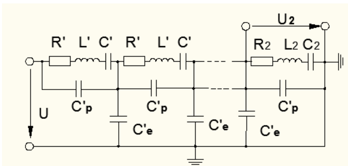
Рис. 8 – Схема заміщення ємнісного дільника
