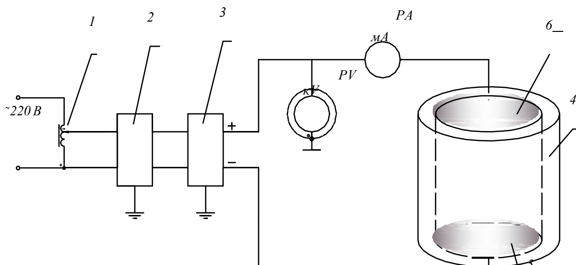
Рис. 1 — Дослідна установка: 1 — автотрансформатор; 2 — підвищувальний трансформатор; 3 — каскадний двополярний помножувач напруги; 4 — циліндр із діелектричного матеріалу; 5 — нижній пластинчастий електрод; 6 — верхній пластинчастий електрод.
