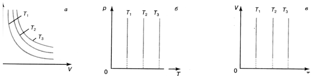
Рис.7. Ізотермічний процес
