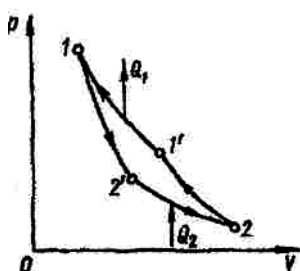
1-1' ізотермічне розширення
