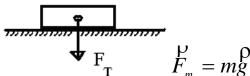
Рис. 2 Сила тяжіння
