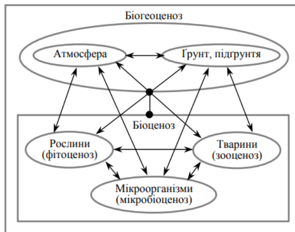
Рис. 6.1. Схема будови біоценозу (за В. М. Сукачовим)
