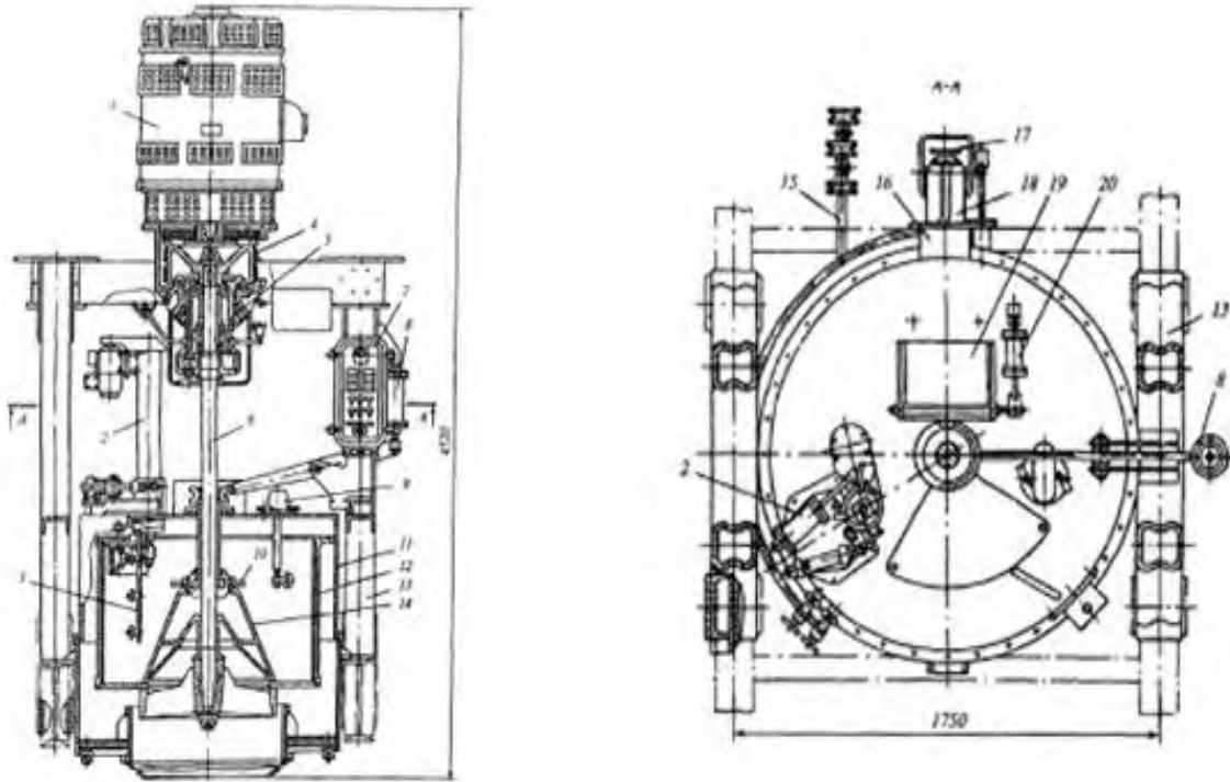
Рис. 2. Центрифуга АПН-1251Л-02
