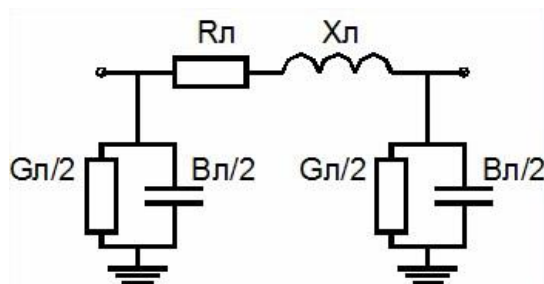
Рис. 40 П-подібна схема заміщення
