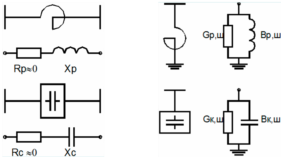
Рис. 42 Схеми індуктивних та ємнісних опорів
