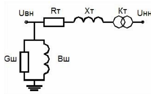
Рис. 41 Г-подібна схема заміщення
