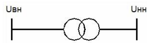
Рис. 41 Схема трансформатора на кресленні
