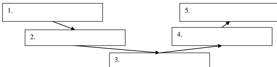
Рисунок 1.1 – Схема документообігу.....
