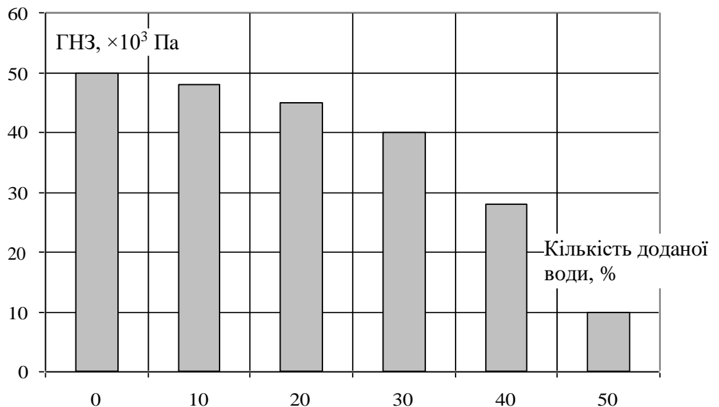
Рис. 2. Залежність граничного напруження зсуву (ГНЗ) горіхової начинки від кількості доданої води
