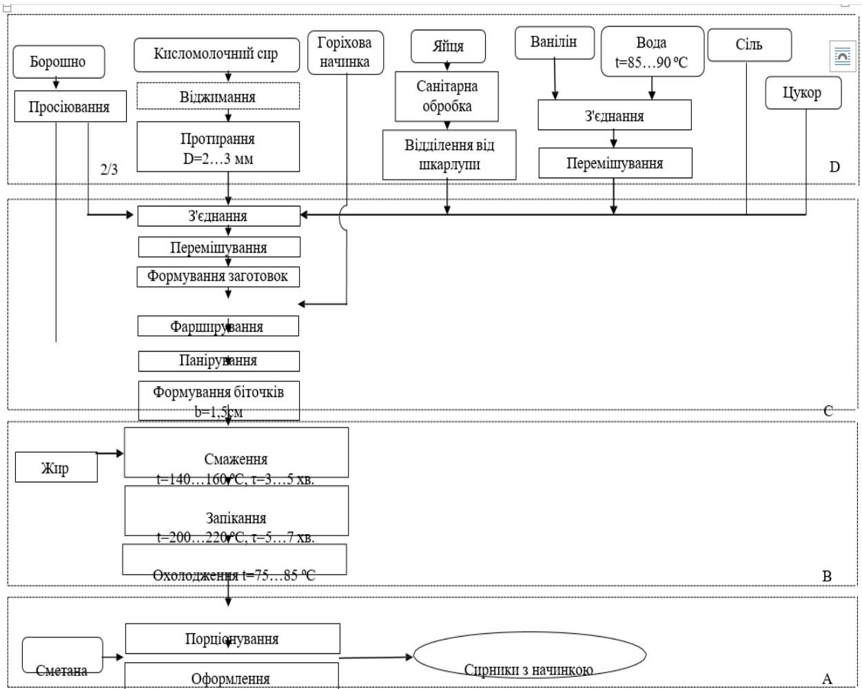
Рис. 1. Технологічна схема виробництва булочки «Звичайної»
