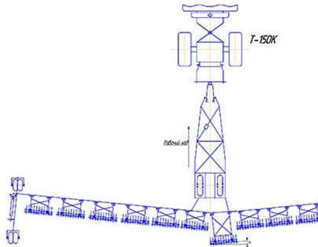
Рисунок 2. Схематичний вигляд лущильного агрегату
