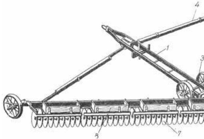
Рисунок 3. Схема луцильника ЛДГ-10. 1 - рама; 2 - брус; 3 - середнє колесо; 4 - тяга; 5 - бокове колесо; 6 - права батарея; 7 - ліва батарея; 8 - баласні ящики.
