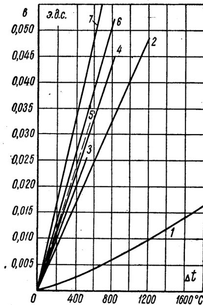
Рис. 4.12 – Залежності термо-е.р.с. від різниці температур спаїв термопар: 1 – платинородій-платина; 2 – хромель-алюмель; 3 – мідь-константан; 4 – залізо-константан; 5 – мідь-копель; 6 – залізо-копель; 7 – хромель-копель
