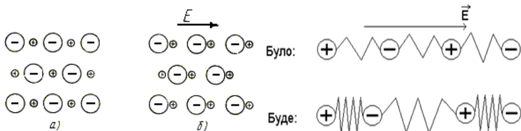
Рис. 8.5 – Схематичне зображення іонної поляризації. Іонна кристалічна решітка: а - при відсутності електричного поля; б - при дії електричного поля
