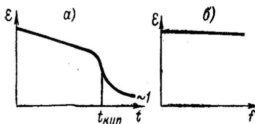
Рис. 8.8 – Залежності діелектричної проникності нейтральної рідини від температури (а) і чистоти струму (б) ( t_{кип} - температура кипіння рідини)
