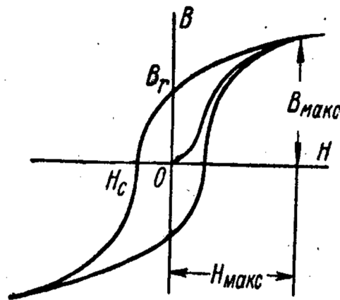
Рис. 16.5 – Початкова крива намагнічування та петля гистерезиса для ферромагнітного матеріалу
