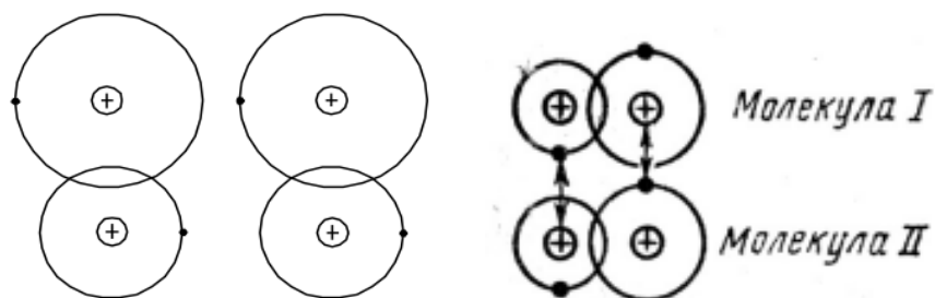
Рис. 1.12 – Схематичне зображення двох взаємодійних молекул (зв'язок Ван-дер-Ваальса)
