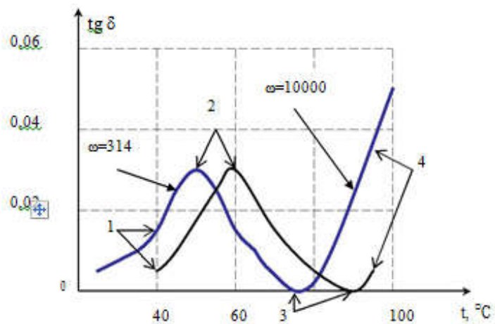
Рис. 10.4 – Залежність діелектричних втрат від температури для масляноканіфольного компаунда
