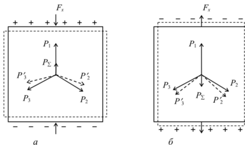
Рис. 3.16 – Деформація стиснення (а) і розтягування (б) пьезоелемента уздовж електричної осі
