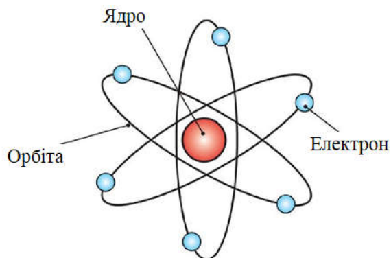
Рис. 1.2 – Планетарна модель атома
