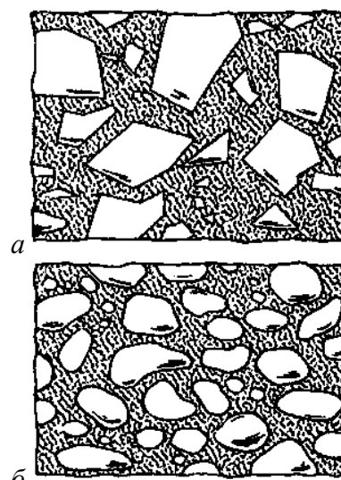
Рис. 6. Брекчія (а) і конгломерат (б)
