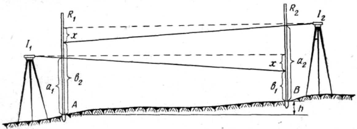
Рис. 3. Перевірка горизонтальності візирного променя
