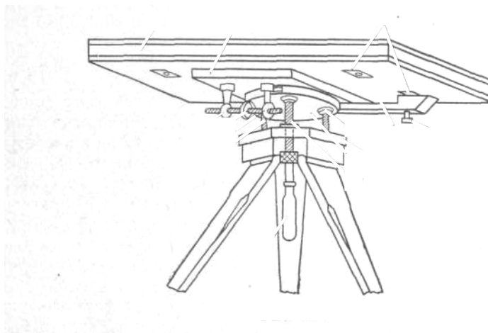
Рис. 11. Мензула
