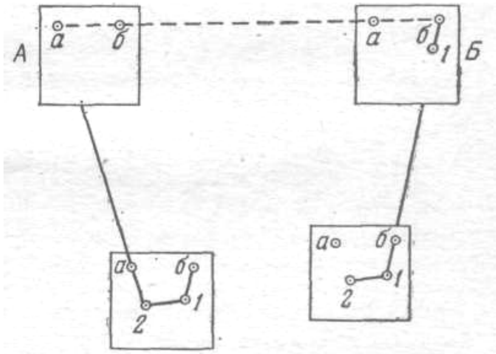
Рис. 22. Прокладання мензурального ходу
