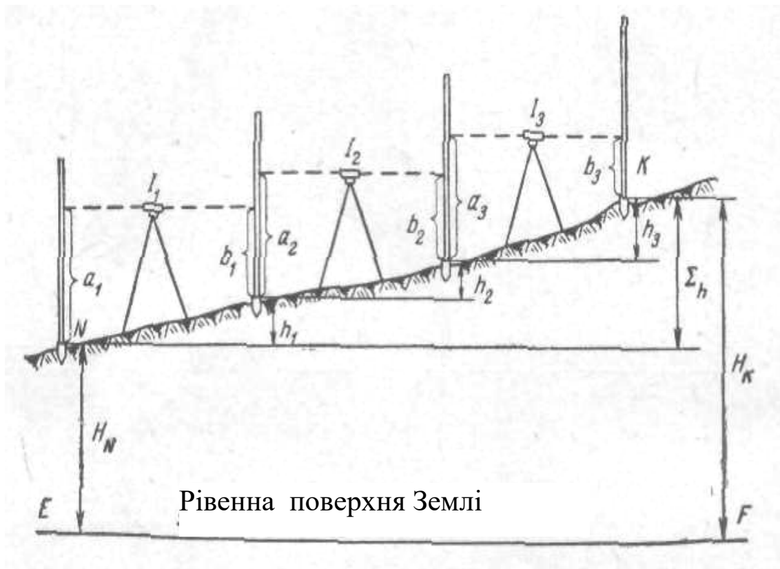
Рис. 7. Складне нівелювання
