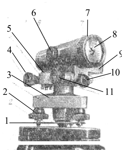
Рис. 1. Будова нівеліра НЗ:
