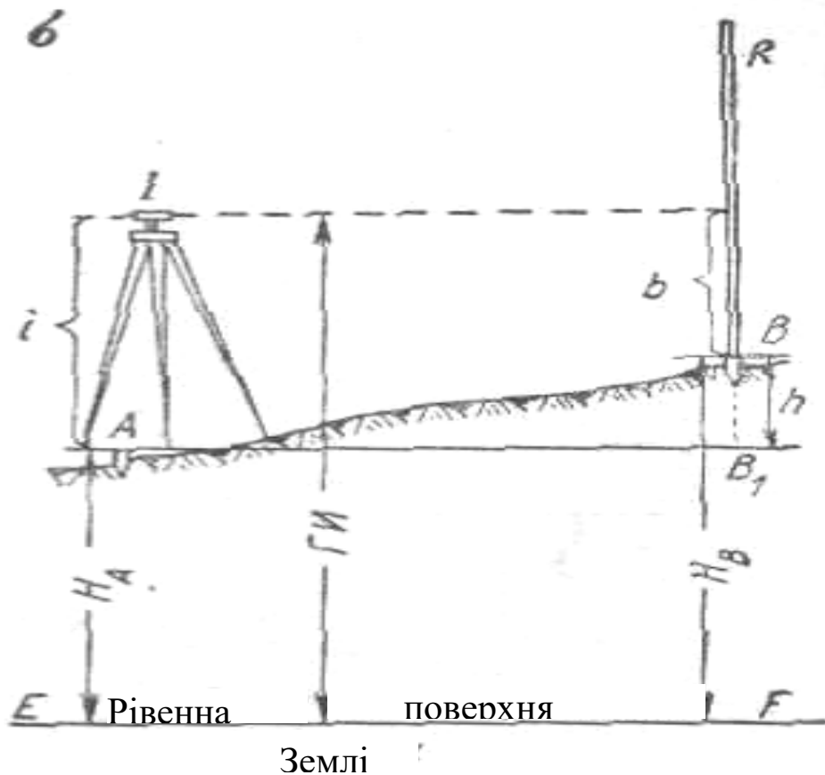
Рис. 6. Нівелювання вперед
