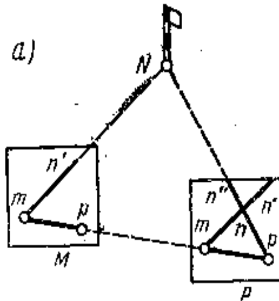
Рис. 19. Прямая засічка
