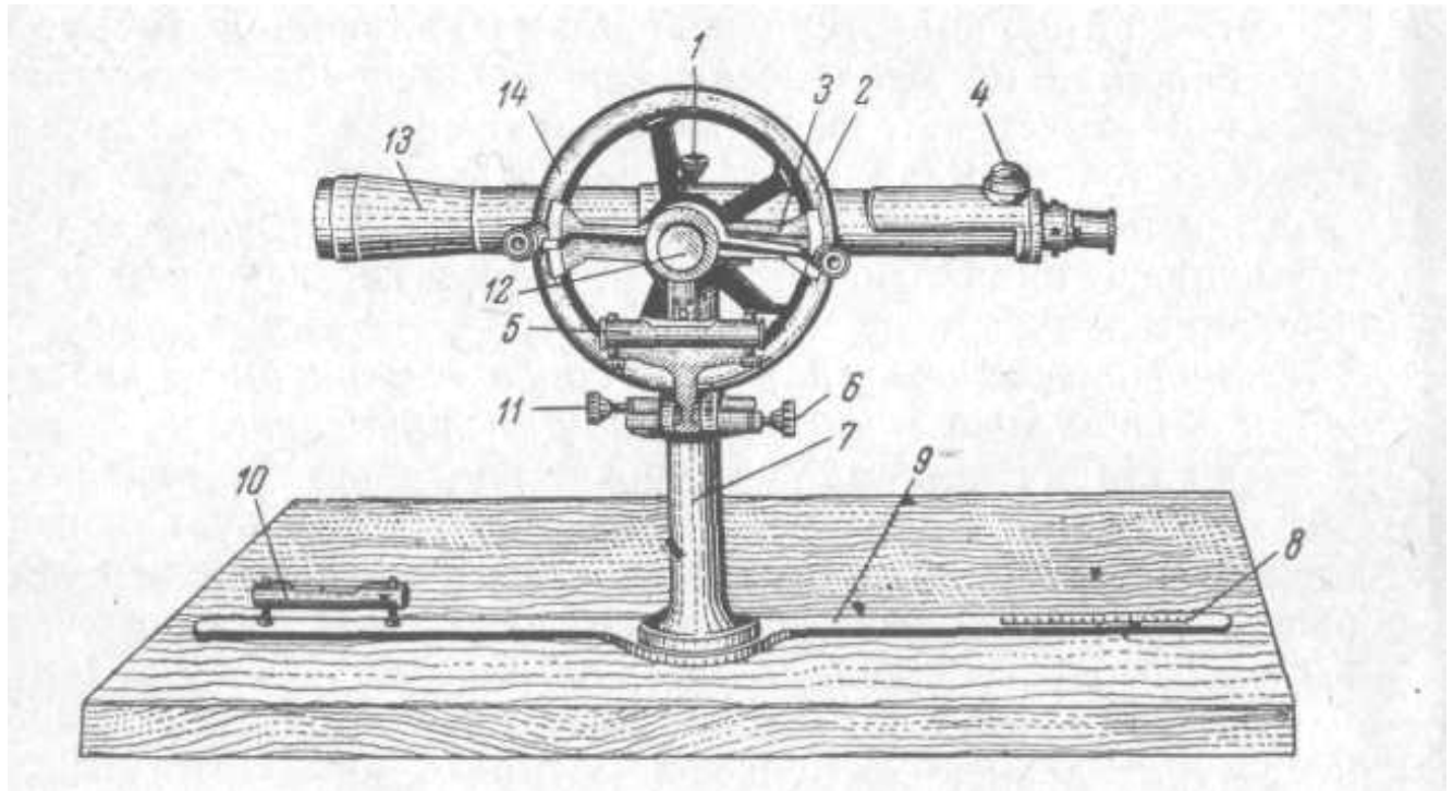
Рис. 14. Кіпрегель
