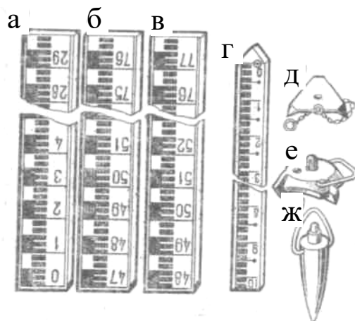
Рис. 4. Нівелірні рейки, башмаки, костилі: а – чорна сторона; б і в – червоні сторони; г – підвісна рейка; д і е – башмаки; ж – костиль
