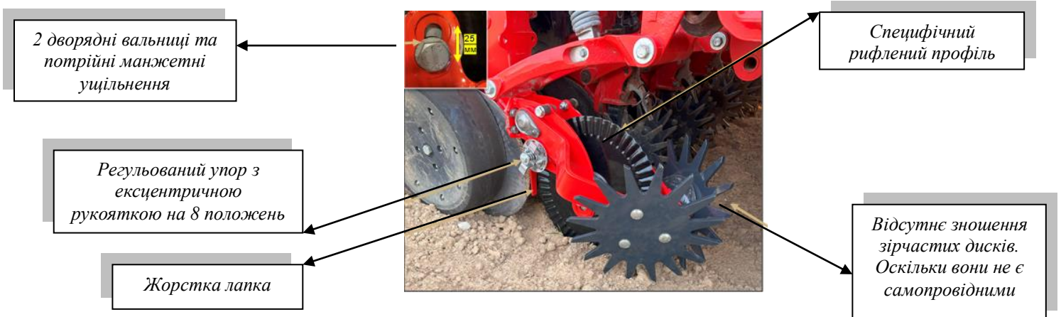
Рис.4.Дисковий сошник із очисником рядків 1
