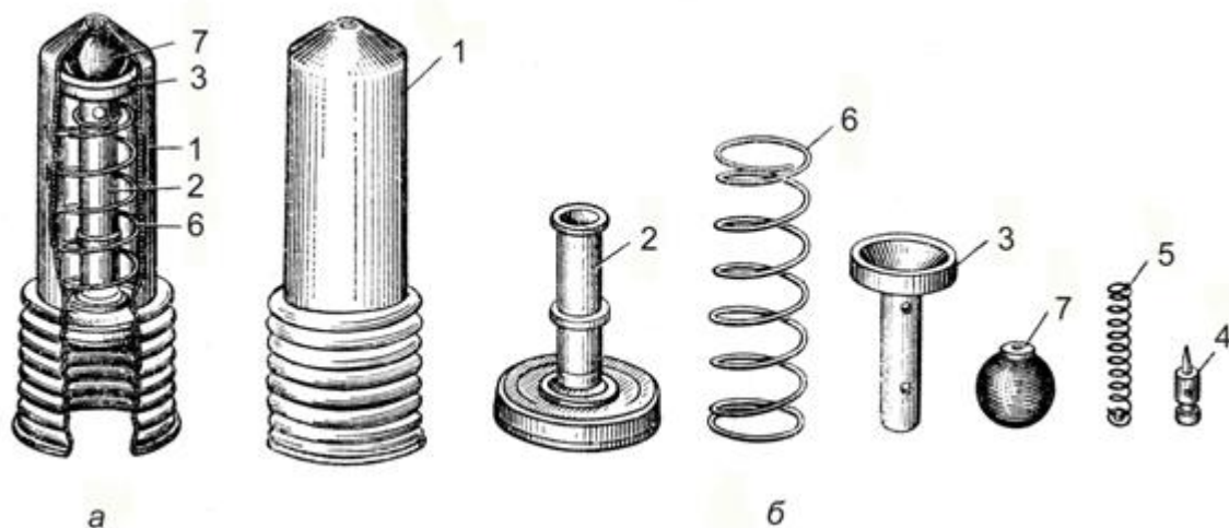
Рис.6. Ударний механізм в розібраному вигляді:
