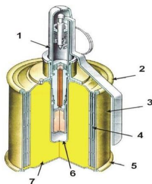
Рисунок – Будова ручної гранати РГ-42
