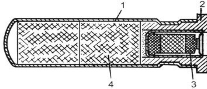
Рис.8. Запал (в розрізі):
