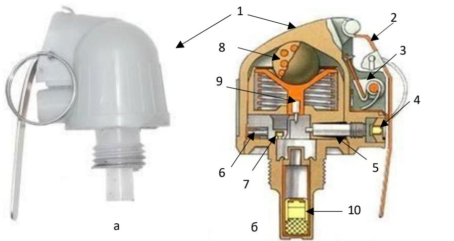
Рисунок – Загальний вигляд та будова ударно-дистанційного запалу.
