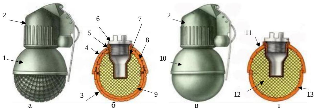
Рисунок – Будова гранати РГО, РГН
