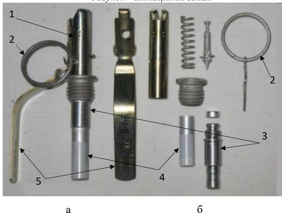
Рисунок – Імітаційний запал.
