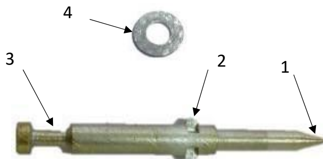
Рисунок – Ударник та шайба ударника
