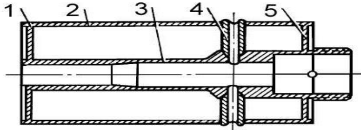
Рисунок – Корпус гранати (в розрізі).
