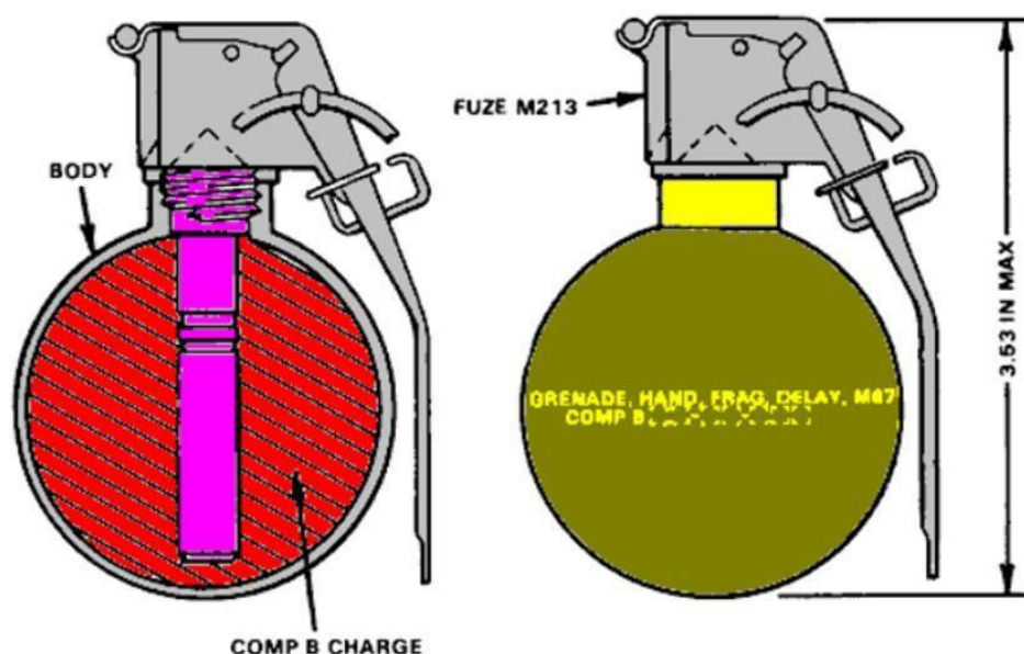
Рисунок – Ручна граната М67 у розрізі.
