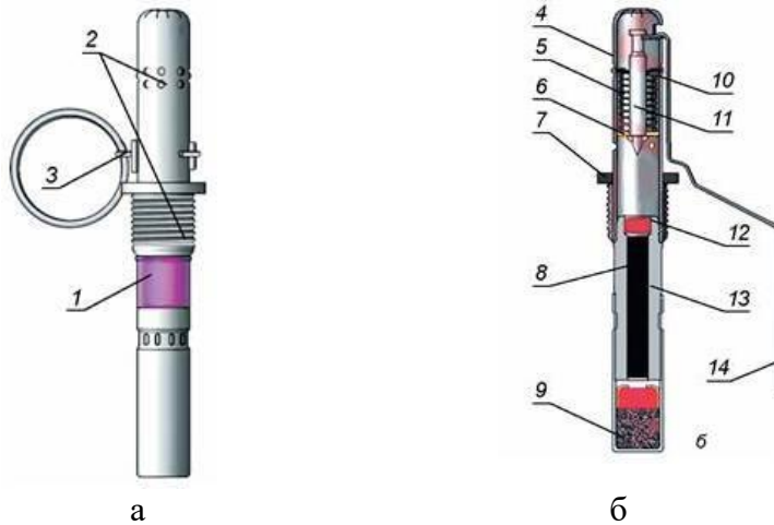
Рисунок – Запал гранати УЗРГМ (УЗРГМ-2)
