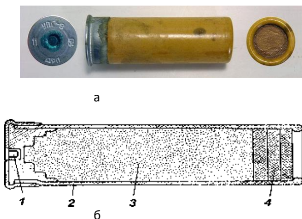
Рисунок – Імітаційний запал гранати УПГ-8.
