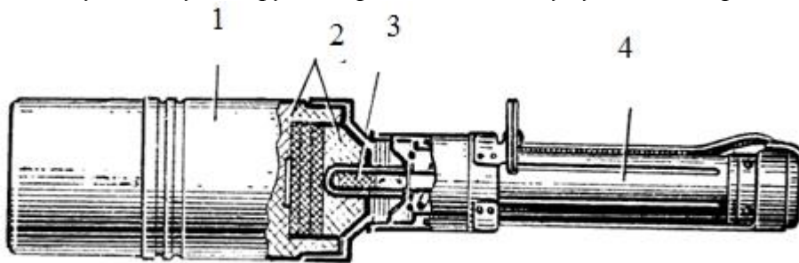
Рисунок – Будова ручної протитанкової кумулятивної гранати РКГ-3
