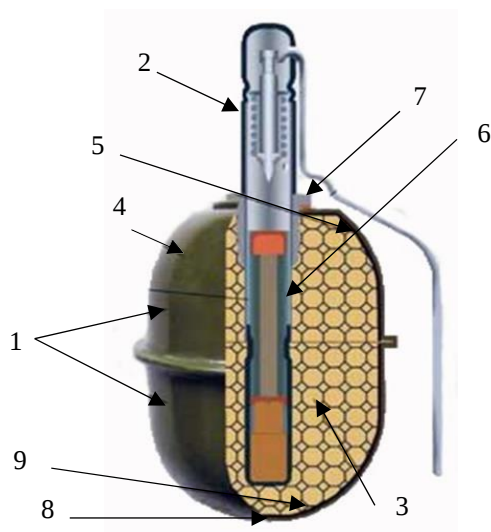
Рисунок – Будова ручної осколкової гранати РГД-5.
