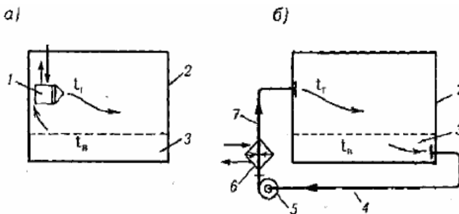
Рис. 14. Схеми повітряного опалення: а — місцева система; б — центральна система; 1 — опалювальний агрегат; 2 — приміщення, що обігрівается (приміщення на рис. 6); 3 — робоча зона приміщення; 4 — зворотний повітропровід; 5 — вентилятор; 6 — теплообмінник (калорифер); 7 — подаючий повітропровід.
