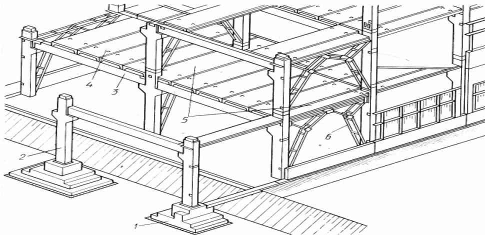
Рис.6. Стійко-балочний рабмий каркас: 1 – фундамент; 2 – колона; 3 – прогін; 4 – настил багатоповерхового перекриття, 5 – зв'язні плити; 6 – вертикальні зв'язки.
