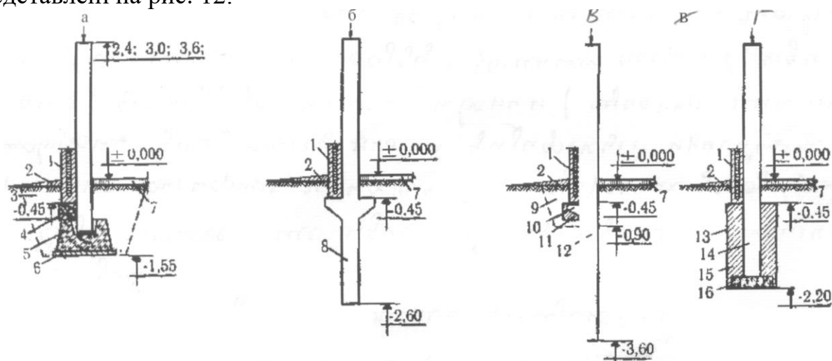
Рис. 12. Елементи фундаментів
