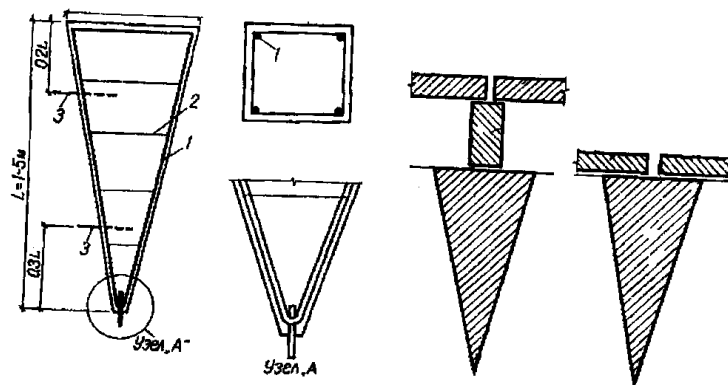
Рис. 11. Розрізи пірамідальних паль
