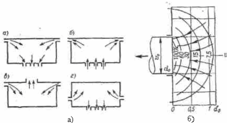
Рис. 17. Схема організації повітрообміну в приміщеннях : а) «зверху – вниз»; б) «знизу – вверх»; в) «зверху – вверх»; г) „знизу – вниз”.
