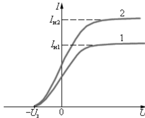
Рис. 31: Залежність сили фотоструму від прикладеної напруги. Крива 2 відповідає більшій інтенсивності світлового потоку. I_{н1} і I_{н2} – струми насичення, U_3 – запираюча напруга.
