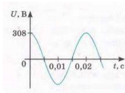
Рис.16. Графік зміни напруги з часом
