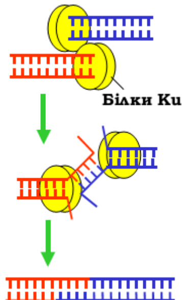
Рис. 36. Негомологічне з'єднання кінців ДНК
