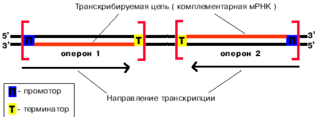
Рис. 3. Синтез молекули РНК
