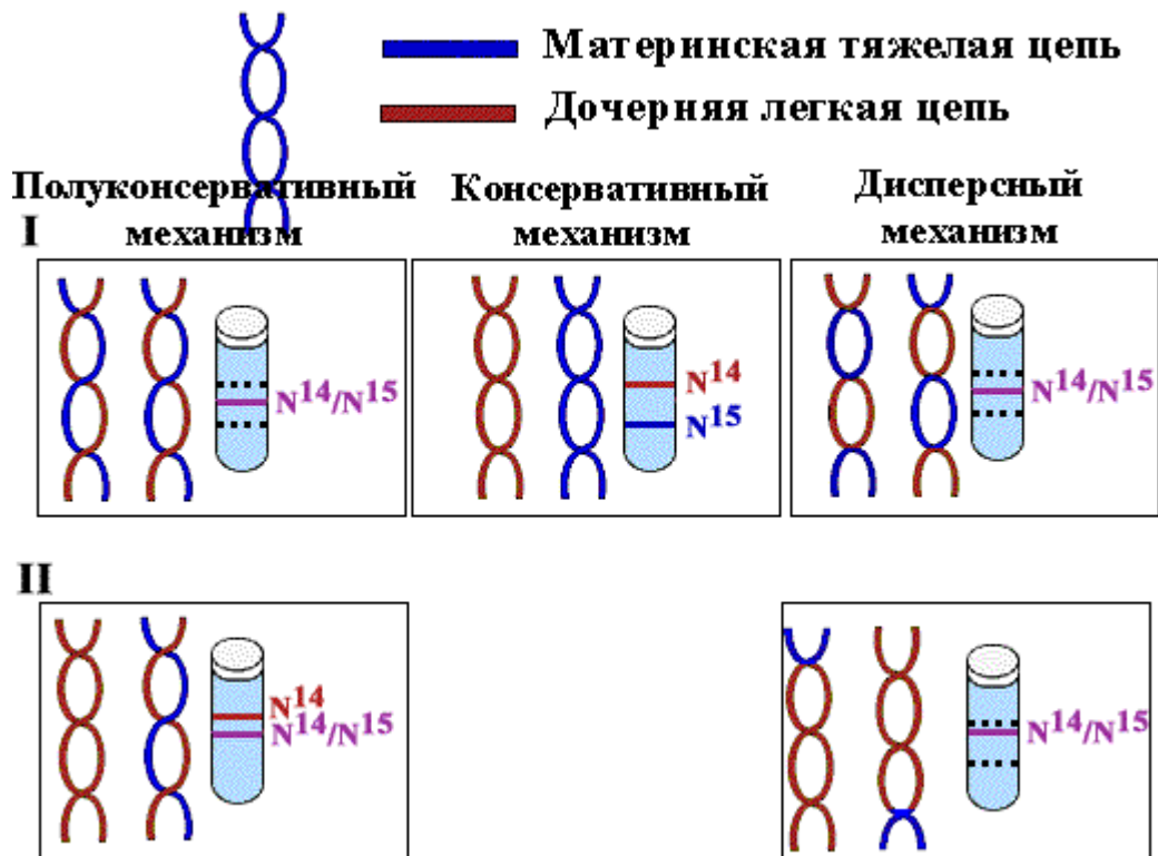
Рис. 14. Гіпотези реплікації ДНК
