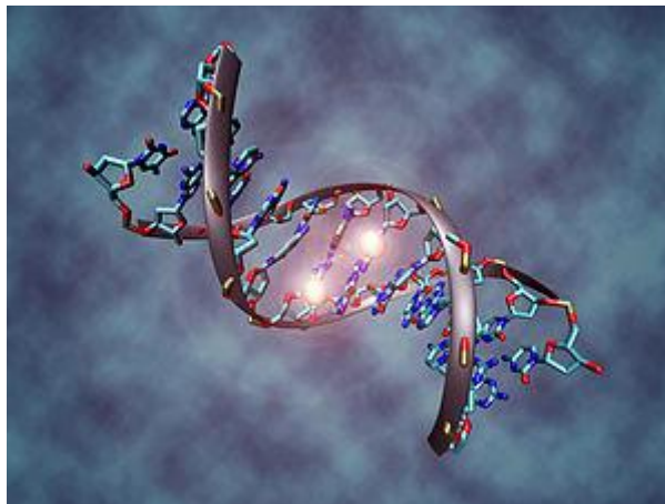
Рис. 17. Ілюстрація молекули ДНК з метильованими цитозинами в центрі.
