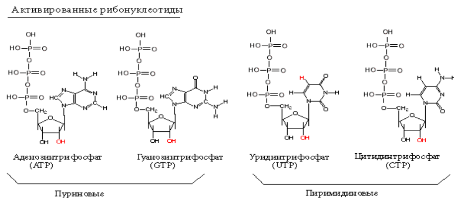
Рис. 2. Активовані рибонуклеотиди
