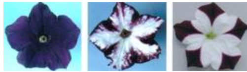
Рис. 37. Квіти Petunia hybrida , в клітинах якої експресія генів, що відповідають за забарвлення знижена РНК інтерференцією.
