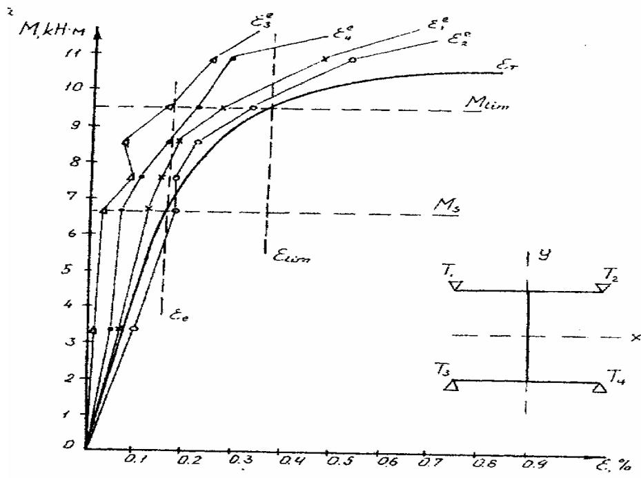
Рис. 1. Експериментальні деформації при одноосному згині бісталевого стержня симетричного перерізу.
