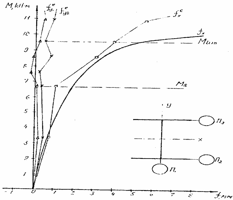
Рис. 2. Експериментальні прогини при одноосному згині бісталевого стержня симетричного перерізу.
