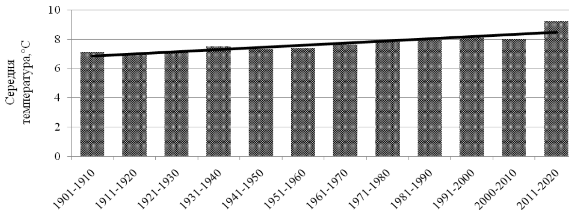
Рисунок 1 – Динаміка зміни середньорічної температури повітря в Україні, 1901-2020 рр.
